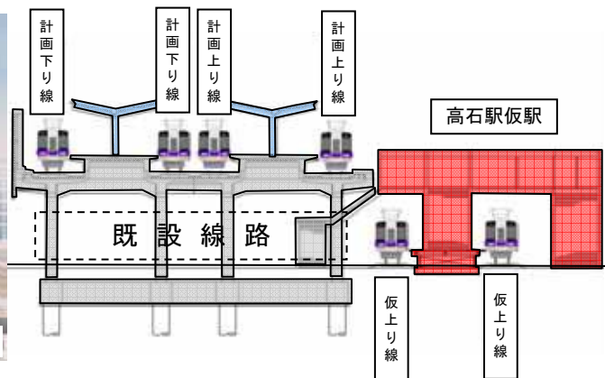
推進費要求箇所断面図
