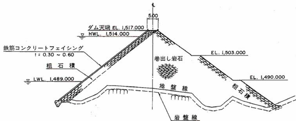
野反ダム標準断面図
