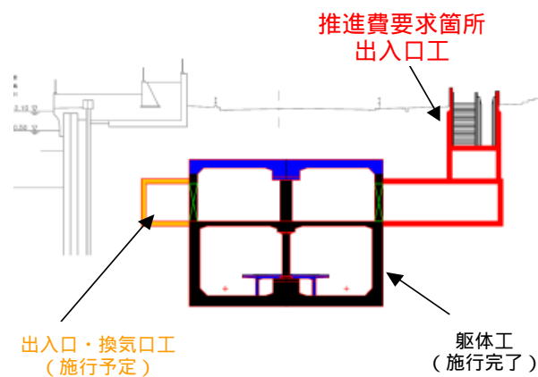
断面図(中之島駅)
