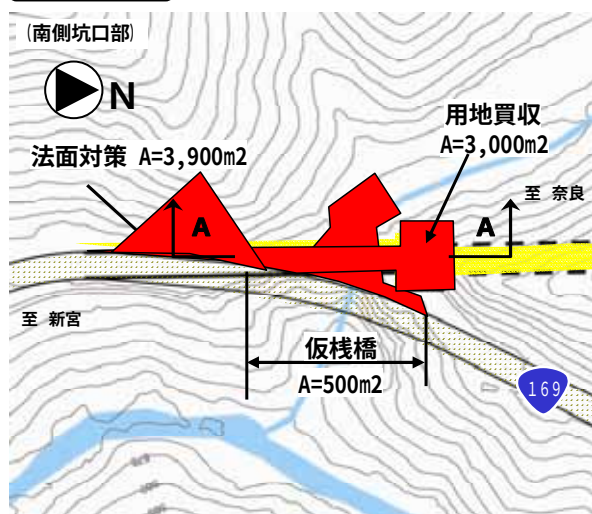
計画図
