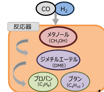
グリーンLPG製造プロセスのイメージ
