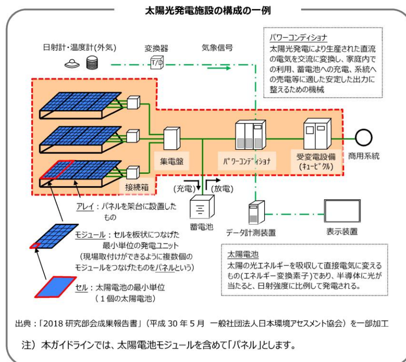
図 4-9 太陽光発電設備の構成の一例
