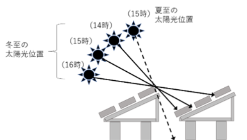
図 4-10 度とパネルの位置関係
