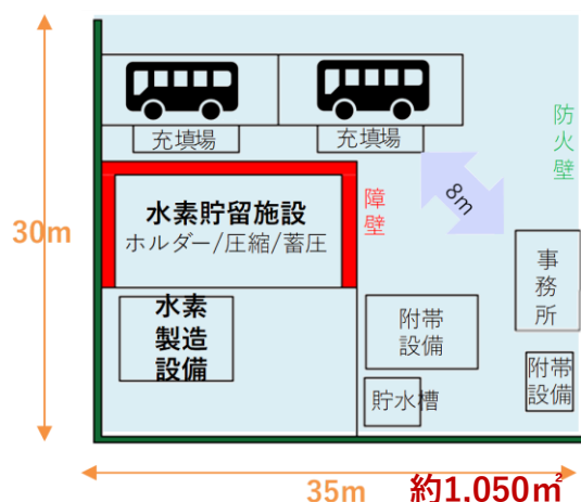
図 3-11 水素ステーション内の施設配置例
