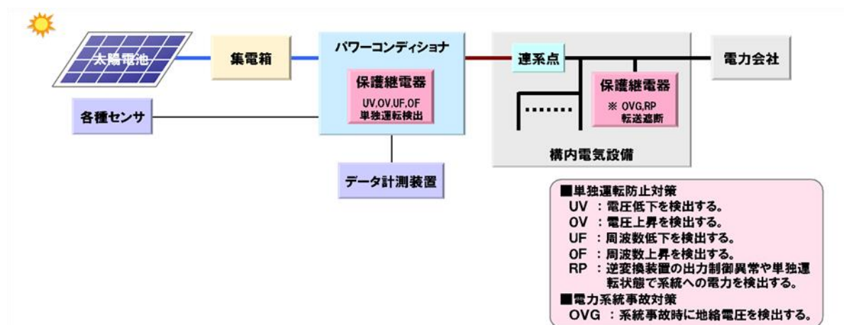
図 4-16 太陽光発電設備の構成
