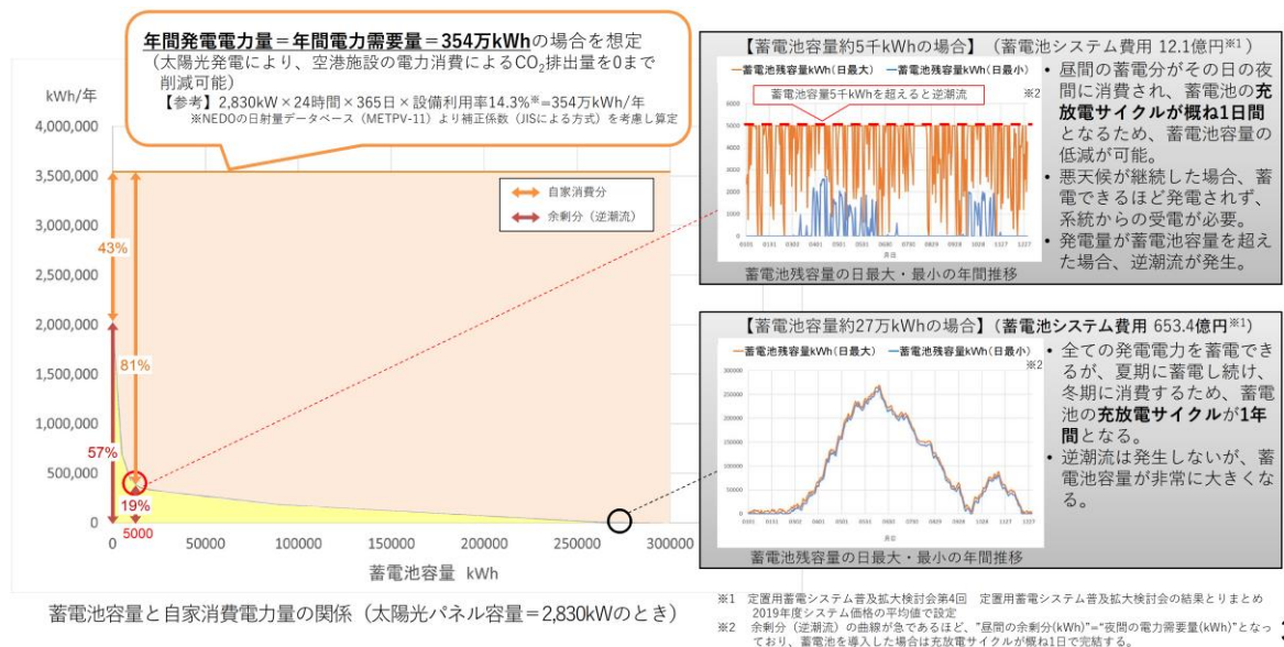
図 4-40 蓄電池の導入検討パターン
