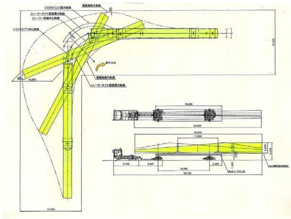
図 4-34 ブレード輸送の検討例
