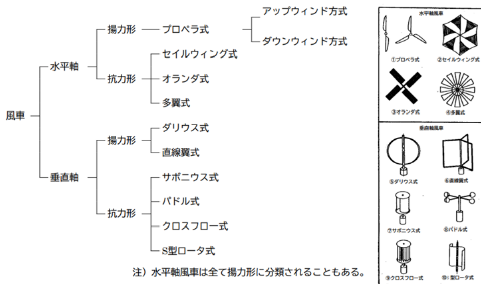
図 4-31 風車の種類
