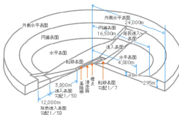
図 4-28 制限表面概略図
