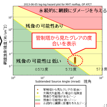
図 4-13 SGHAT による参考シミュレーション
