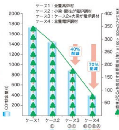
図 2-5 建築鉄骨構造例と電炉鋼材適用による CO2 排出量削減効果
