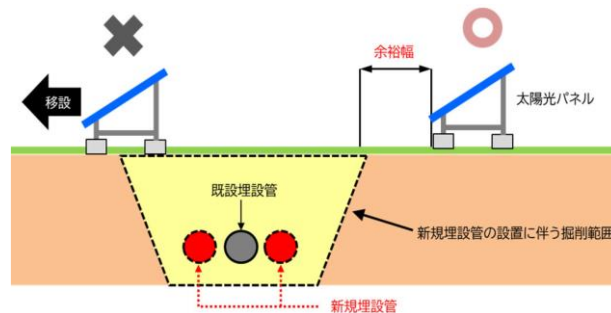
図 4-8 埋設物付近の余裕幅の設定イメージ
