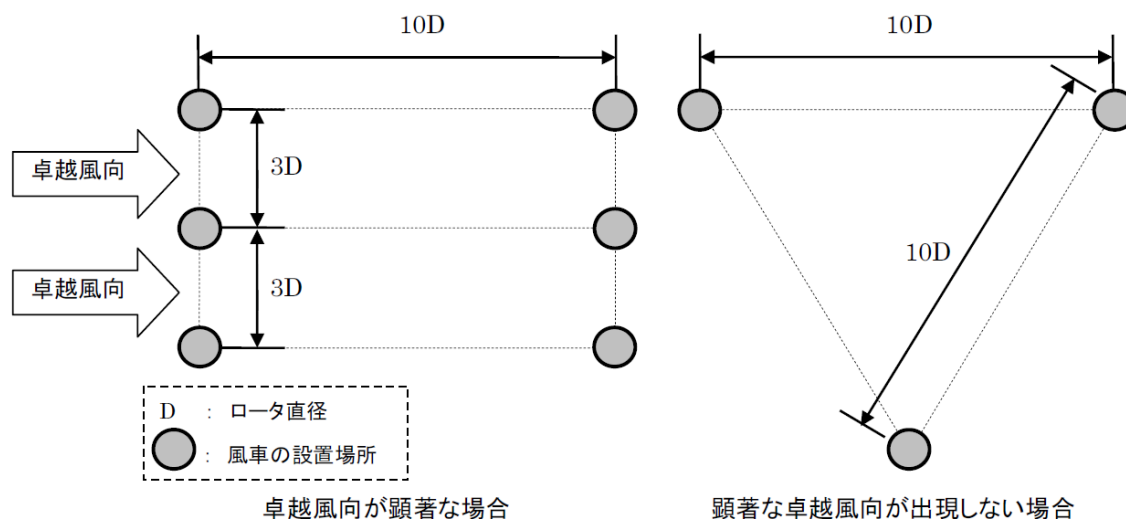
図 4-32 風車の配置方法（複数台設置の場合）
