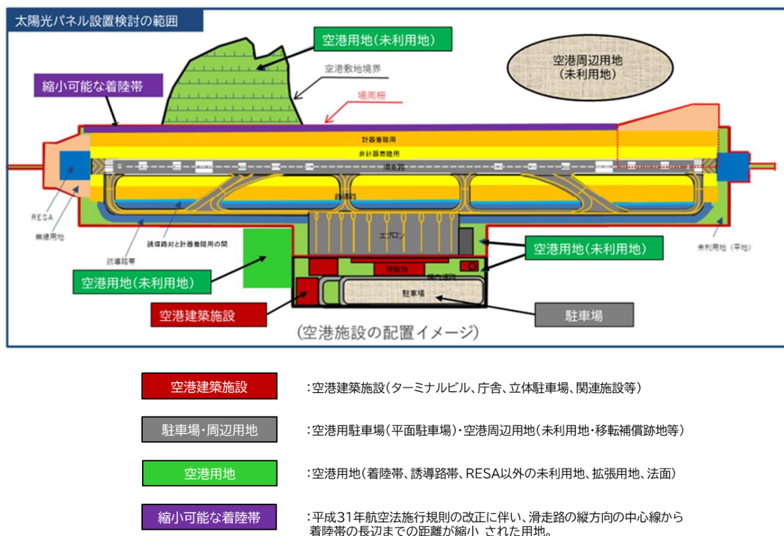
図 4-5 太陽電池パネルの設置検討の範囲
