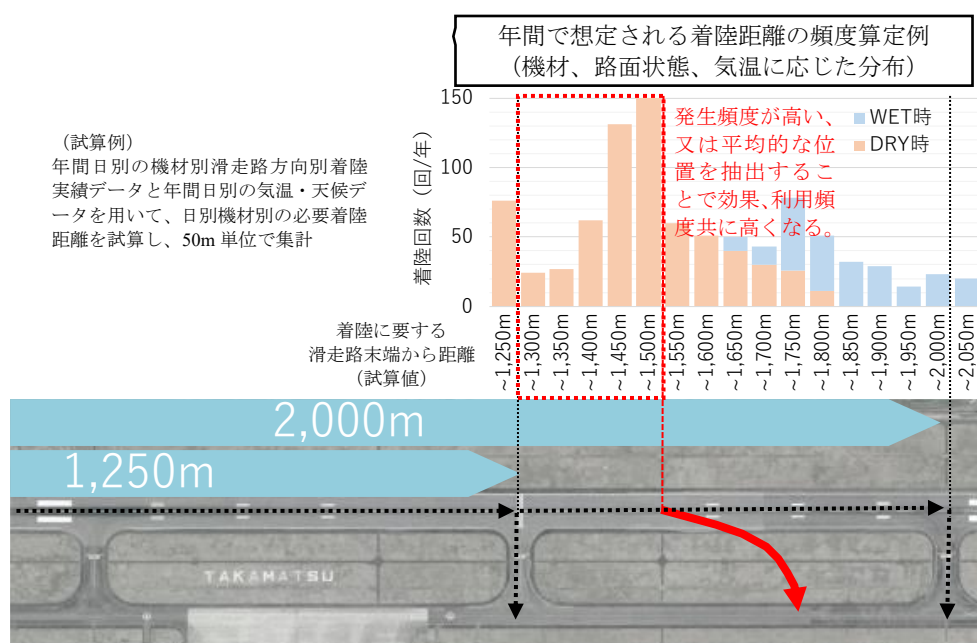
図 5-9 通年の気候を踏まえた必要離着陸距離の分布例
