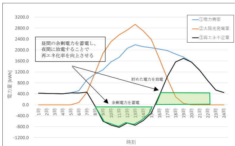
図 4-11 電力需給シミュレーション例
