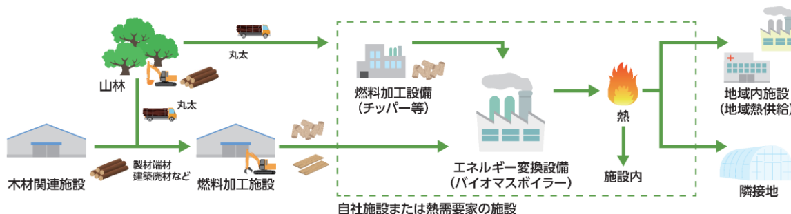
図 4-35 木質バイオマスの事業モデル
