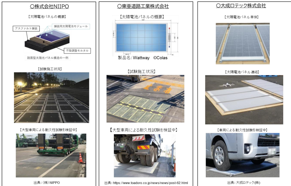
図 4-21 路面型太陽電池の試験事例
