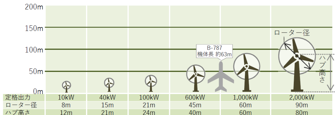
図 4-29 風車の規模と発電出力の関係
