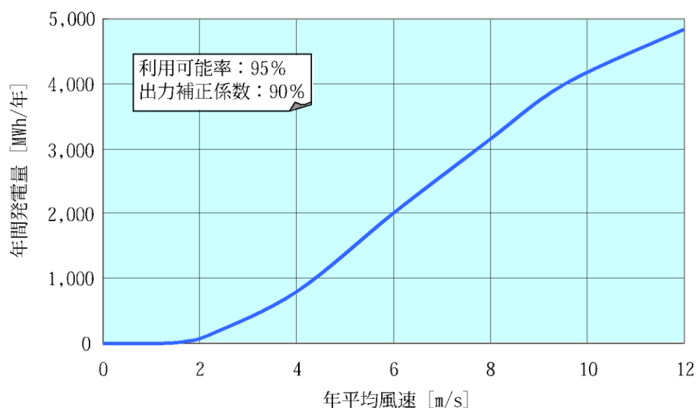
図 4-24 年平均風速と年間発電量の例（出力 1000kW の風車を設置した場合）
