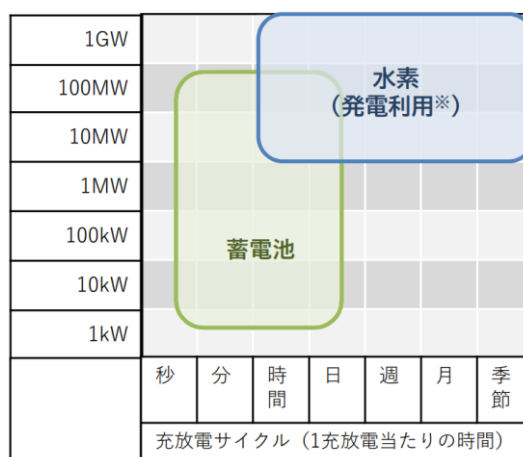
図 4-44 水素（発電利用）と蓄電池の比較
