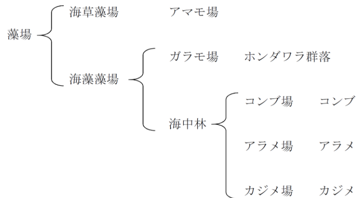
図 7-15 藻場の分類（概要）
