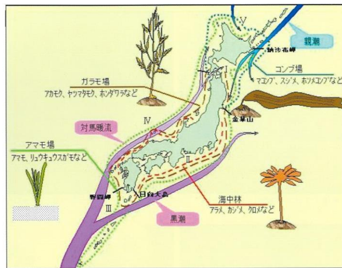
図 7-15 藻場の分類（概要）
