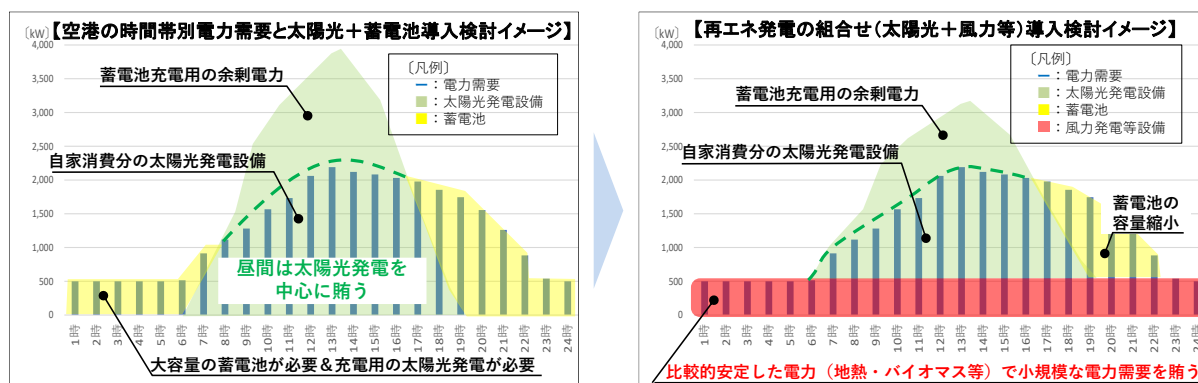
図 6-6 複数の再エネ発電システムの組み合わせによる再エネ化率向上のイメージ
