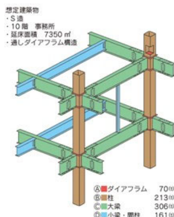
図 2-5 建築鉄骨構造例と電炉鋼材適用による CO2 排出量削減効果
