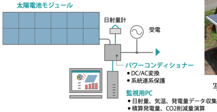
図：太陽光発電設備構成図
