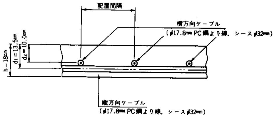
付図-10.1 PC 鋼材の位置の標準
