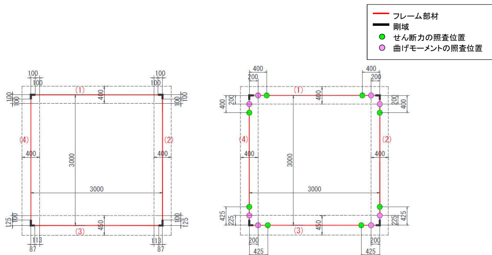
例図-4.10 構造解析モデル（フレーム）
