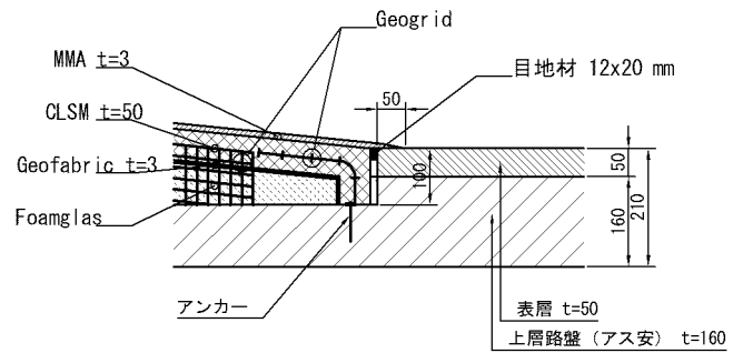
A-A断面図
