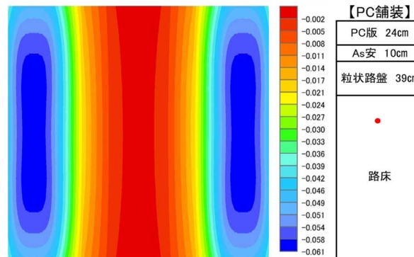
付図-2.6 NC (24cm) 舗装下部 深度 100cm 最大応力 : 60.6kPa
