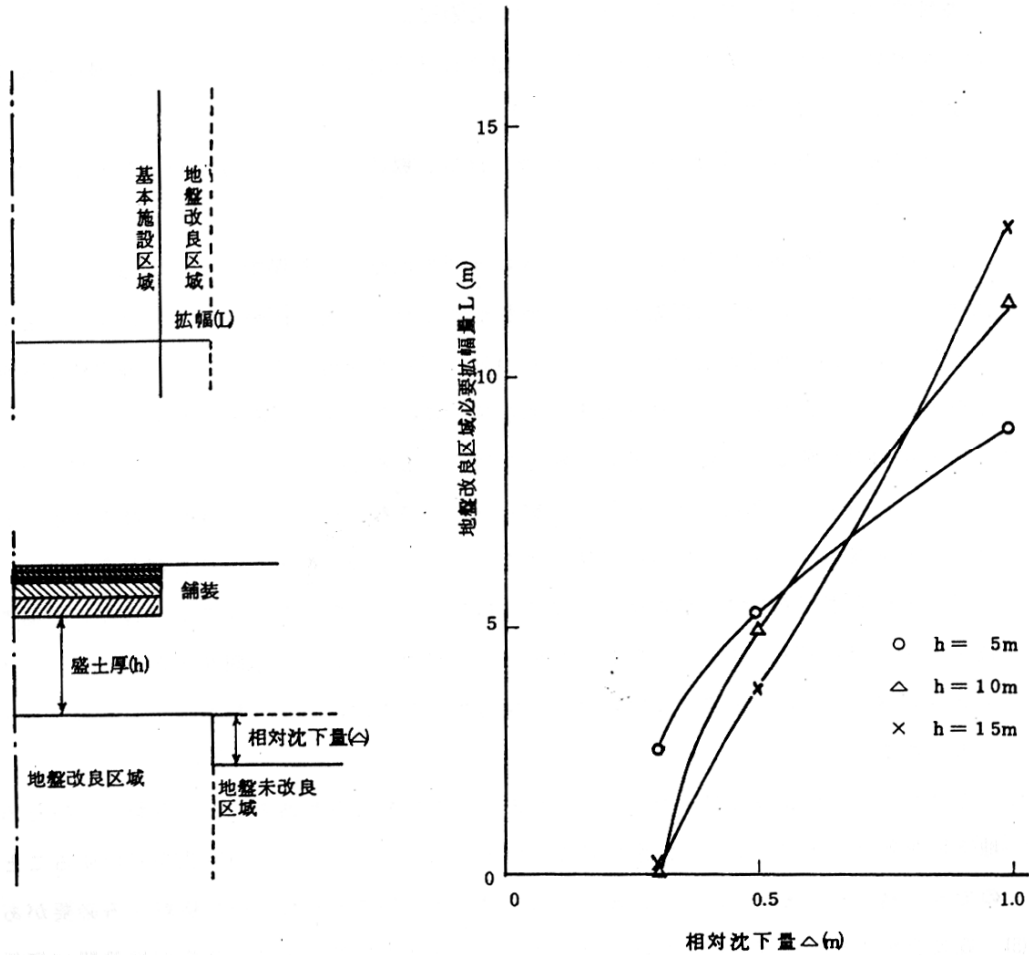
例図-3.1 地盤改良区域拡幅必要長の検討例
