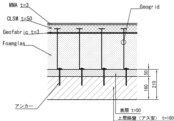
標準構造図
