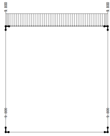
躯体自重
