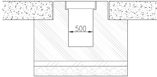
付図-4.5 U型側溝の構造寸法
