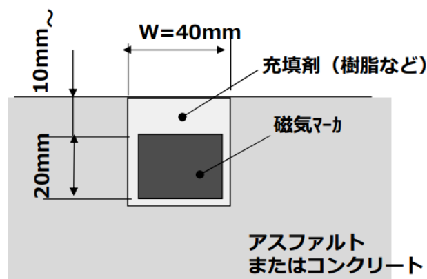
図 3.1-3 磁気マーカーの設置深さ（溝掘削の場合）
