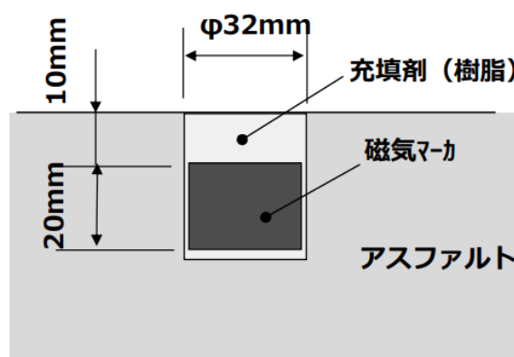
図 3.1-2 磁気マーカーの設置深さ（孔掘削の場合）
