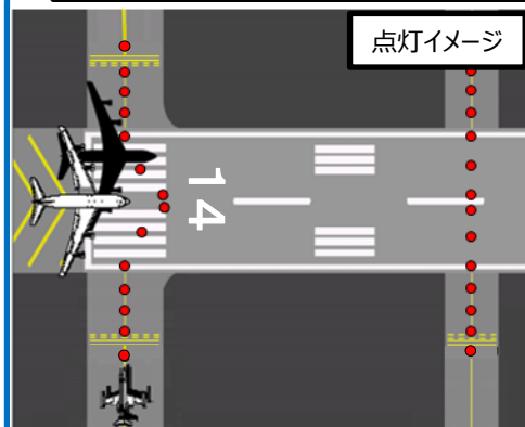
航空機接近警告灯（REL）
