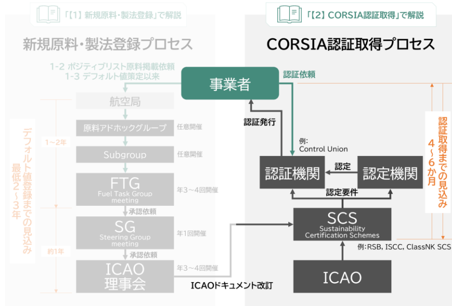
図7 CORSIA 認証取得プロセス
