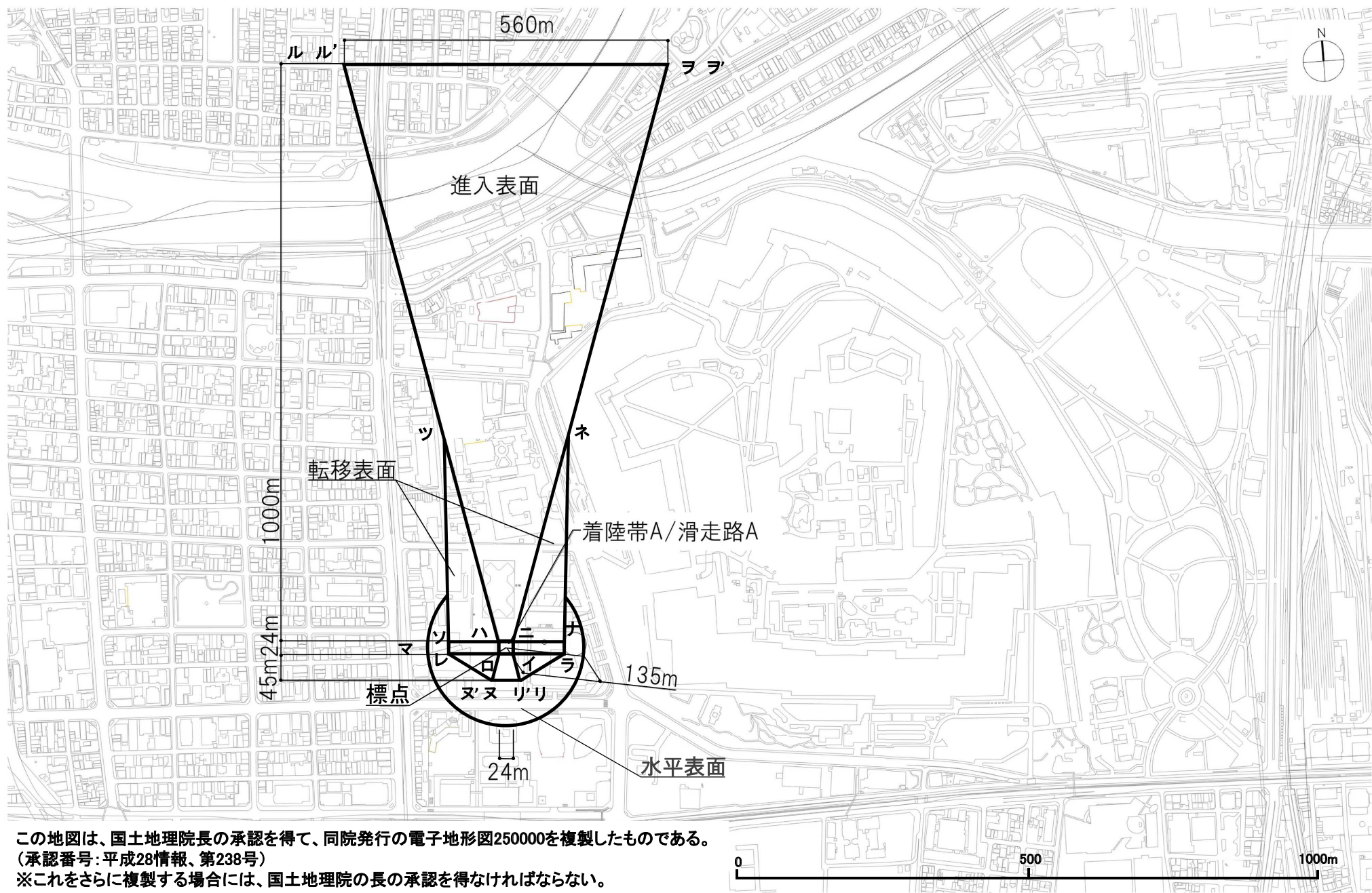
第二図 近畿地方整備局屋上ヘリポート
