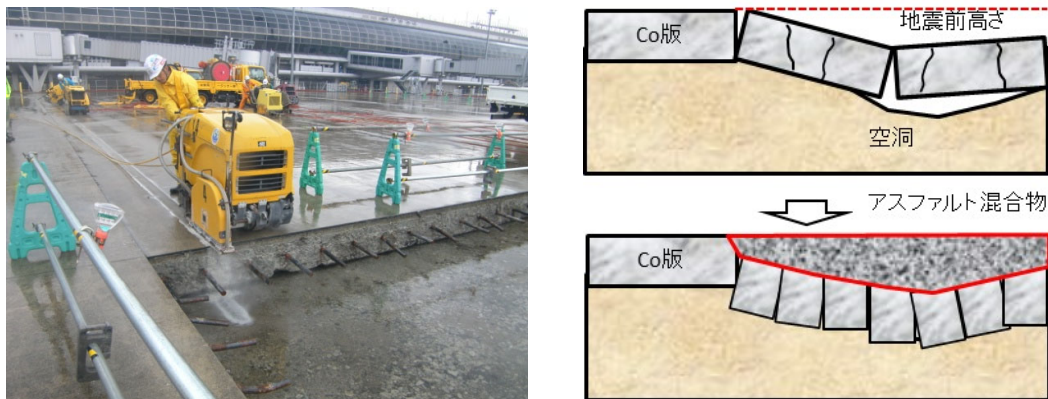
図ー4. 3 ブロック状に切断する応急復旧の例（2011 年仙台空港）
