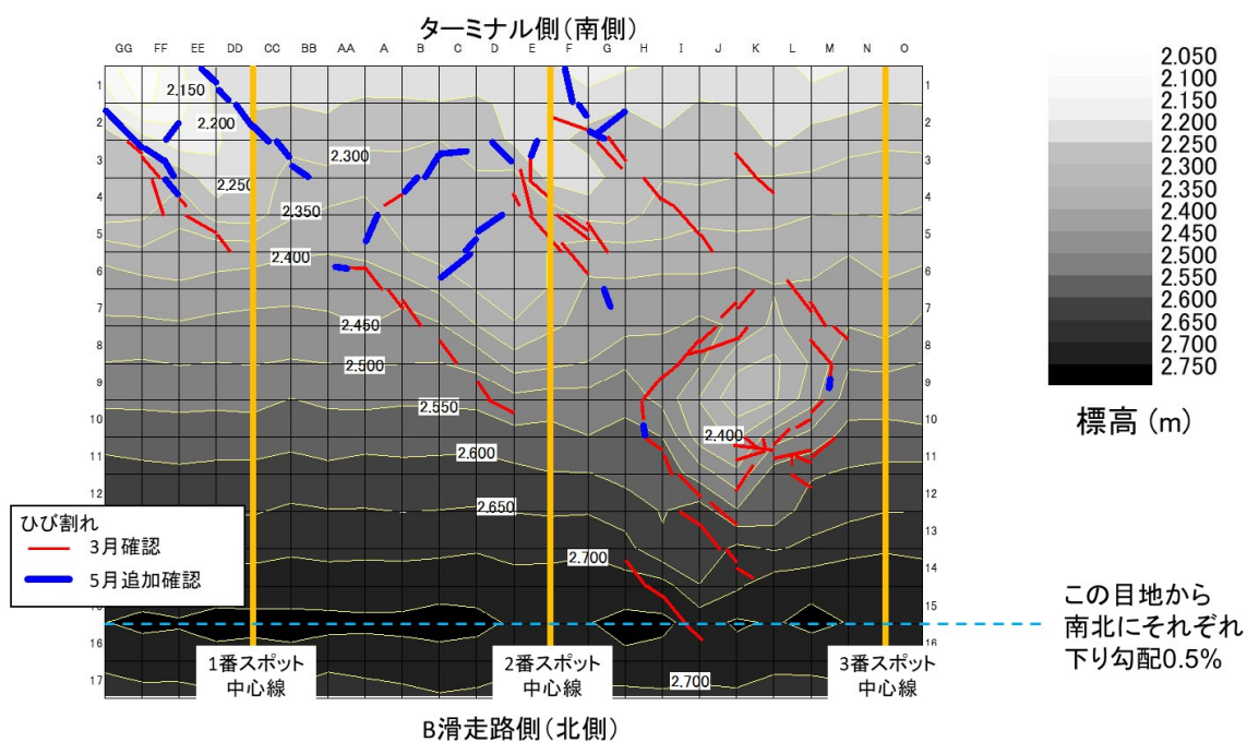
図－3. 4 エプロン（コンクリート舗装）における局所沈下の例（2011 年仙台空港） （升目は1枚のコンクリート版（7.5m×7.5m）である）
