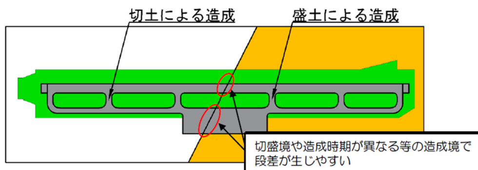
図－２．２ 【段差を有するひび割れ】が懸念される箇所の例
