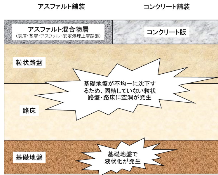
図－3. 1 想定される空洞
