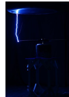
昨年度の雷撃試験の様子 (2025年2月 (株)昭電 テクノセンター)
