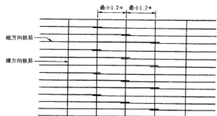
(2) ちどり型
