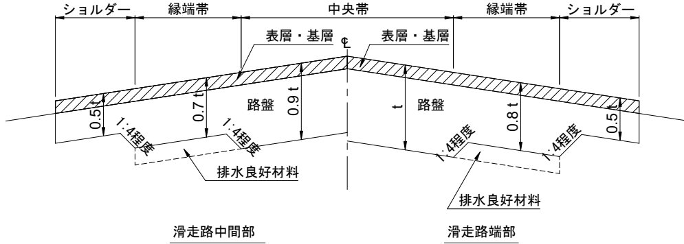
付図-7.2(1) 基準舗装厚の減厚（断面）
