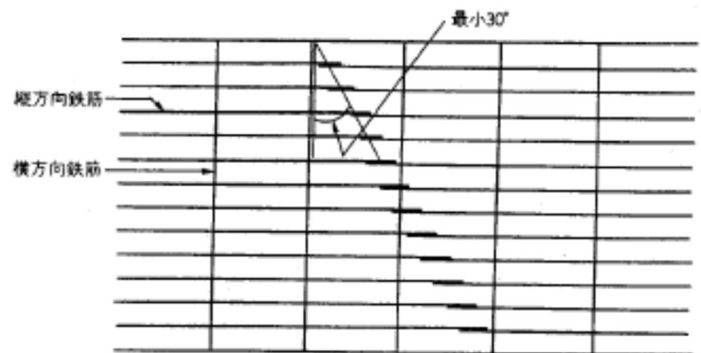
(4) 斜め型
