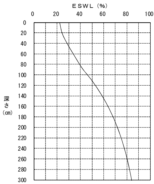
例図-1.13 B777-200
