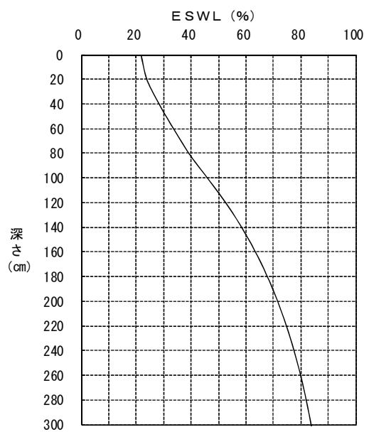
例図-1.16 B777-300ER
