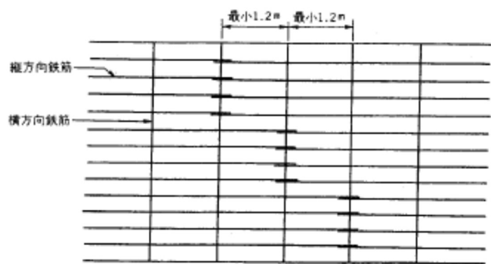
(1) ちどり型
