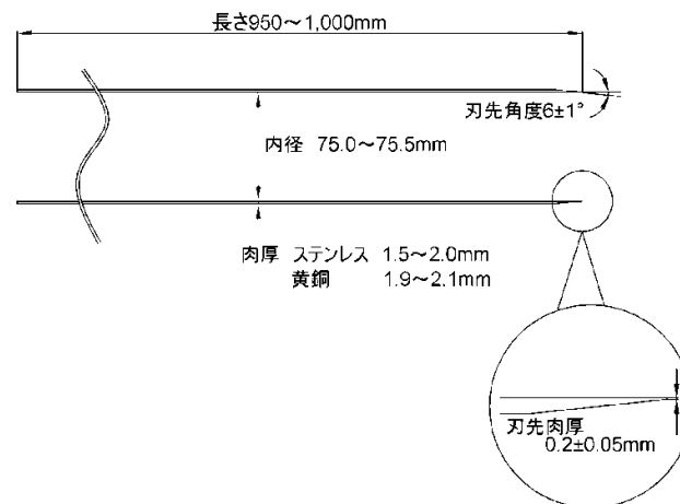
図3-1 サンプリングチューブ
