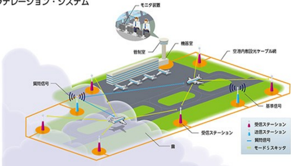
マルチラレーション・システム
