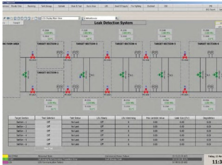
間接検知システム監視画面
