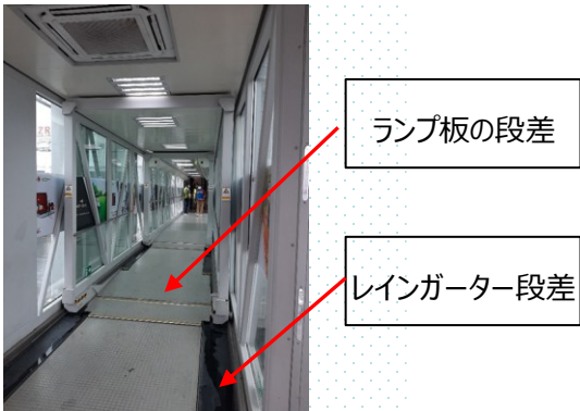
既存PBBトンネル内の段差
