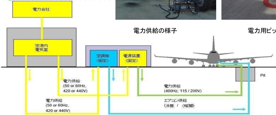
埋設型GPU/PCAシステム 概要図
