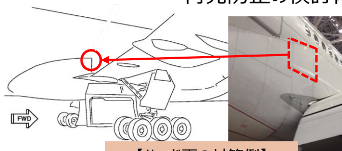
【ハード面の対策例】 機体の改修
