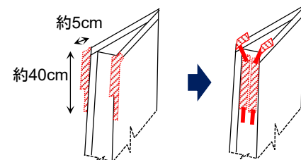
改良前の避雷板
