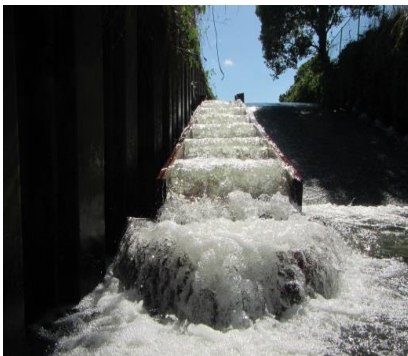
2019年度に設置した際の魚道
