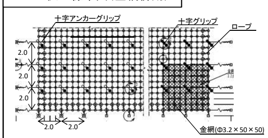
ロープ伏工標準図(金網併用)
