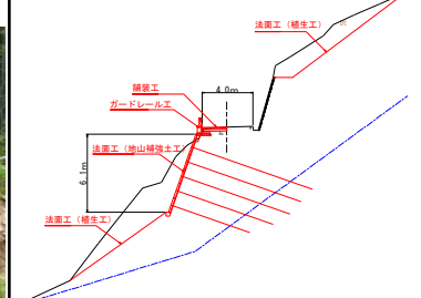
【断面図】A-A'断面
