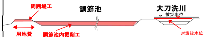
【断面図】 A-A' 断面
