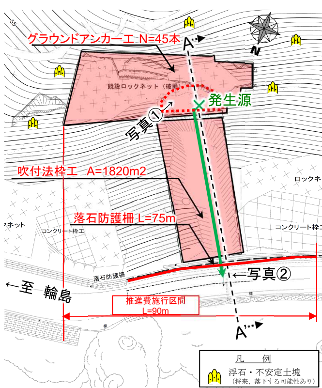
【平面図】
