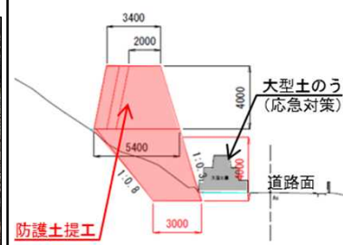
【断面図】A-A'断面
