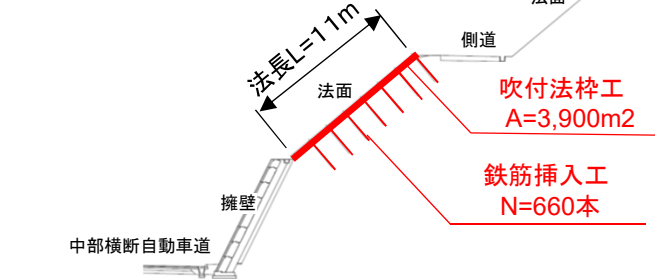
【断面図】A-A'断面
