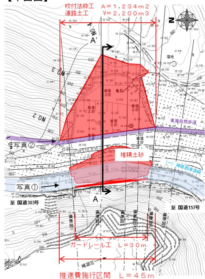
【平面図】
