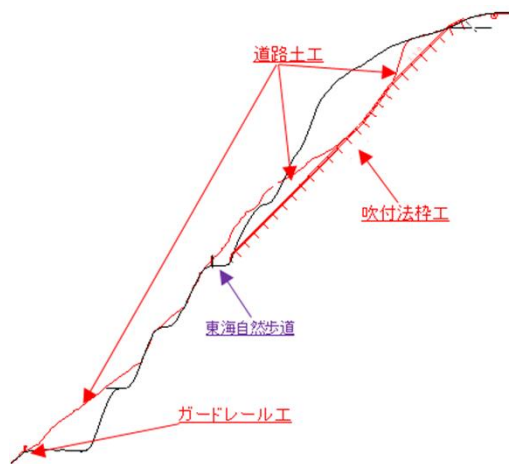
【断面図(A-A')】
