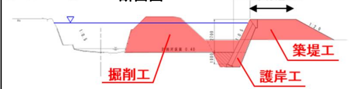
【断面図】 A-A'断面図
