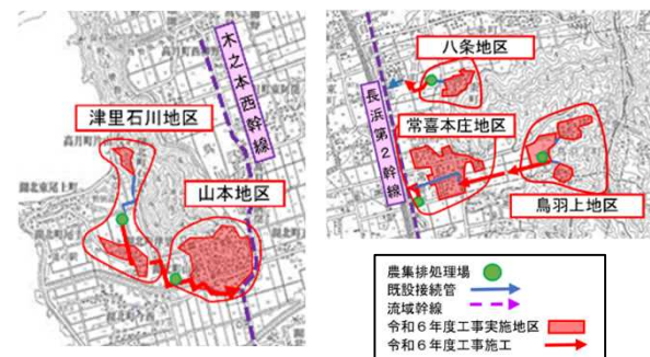
農業集落排水の統合(長浜市)
