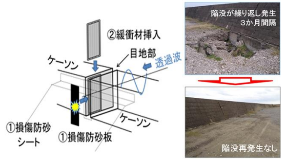
ケーソン目地透過波低減法の概念図(右写真は適用事例)
