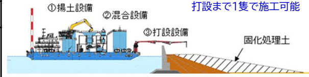
図1 施工イメージ図
