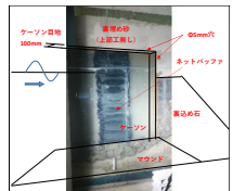
現地1/4実験模型(港湾空港技術研究所)
