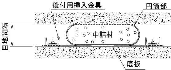
図1 取付概略図
