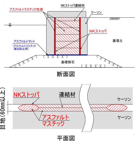
図-1 NKストップパ施工例(ダブルタイプ)
