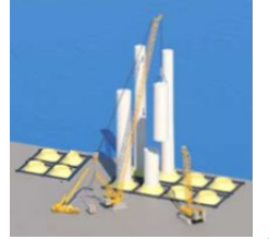
風車資材荷降ろし／保管／プレアッセンブリ
