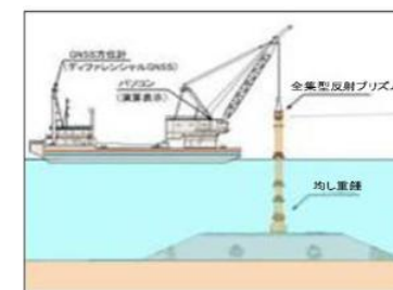
機械均し機の施工管理システムから施工履歴データ取得イメージ
