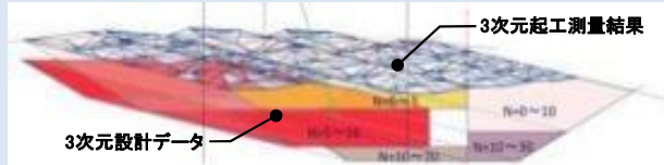
3次元起工(測量結果と3次元設計データから正確な施工量(床掘・置換量)を算出)
