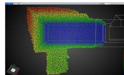
点群より作成した出来形管理図表の例
