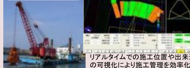
【施工箇所の可視化】
