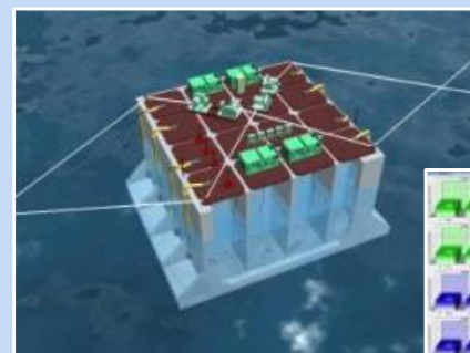
【ICT本体工】 ケーソンの半自動据付
