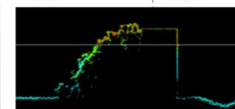
グリーンレーザ&マルチビーム合成断面事例
