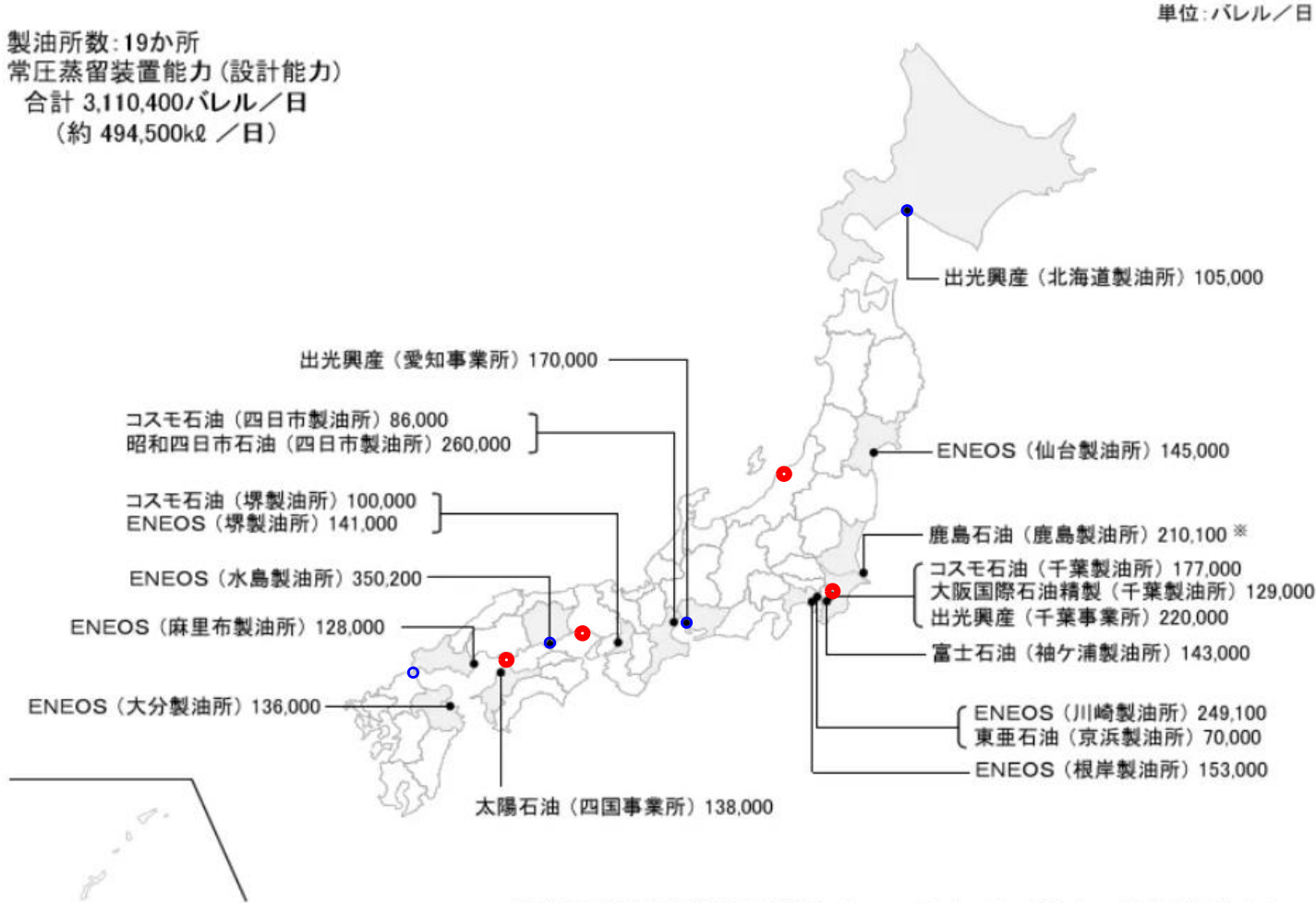
製油所の所在地と原油処理能力 (2024年7月末現在)
