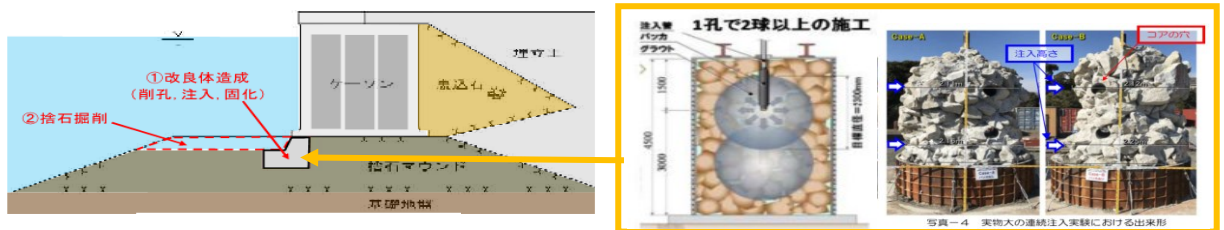
可塑状グラウト増深工法 イメージ
