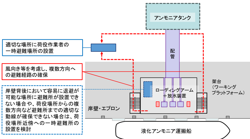
図-5.7 避難所の設置イメージ
