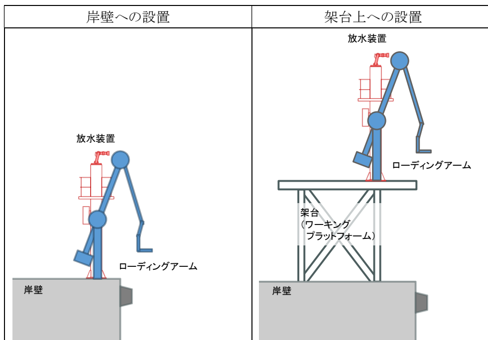
図-5.6 荷役設備の構造例
