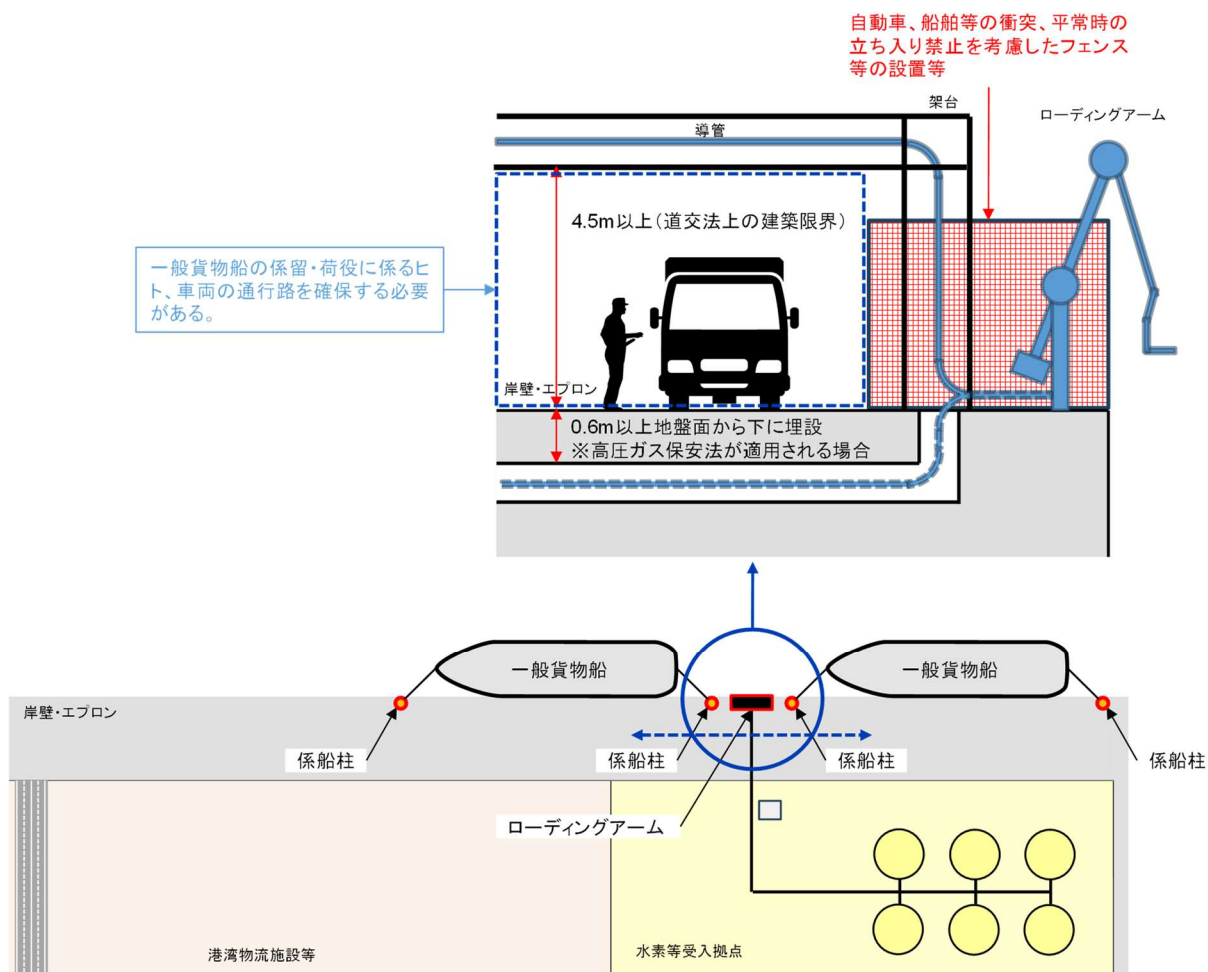
図-5.8 他船舶の係留、荷役に係るヒトや車両に配慮したパイプラインの配置のイメージ
