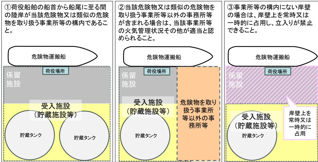
資料：海上保安庁「危険物専用岸壁（D岸壁）の基準等」を基に作成 図-2.4 危険物専用岸壁（D岸壁）の基準等における事業所との関係
