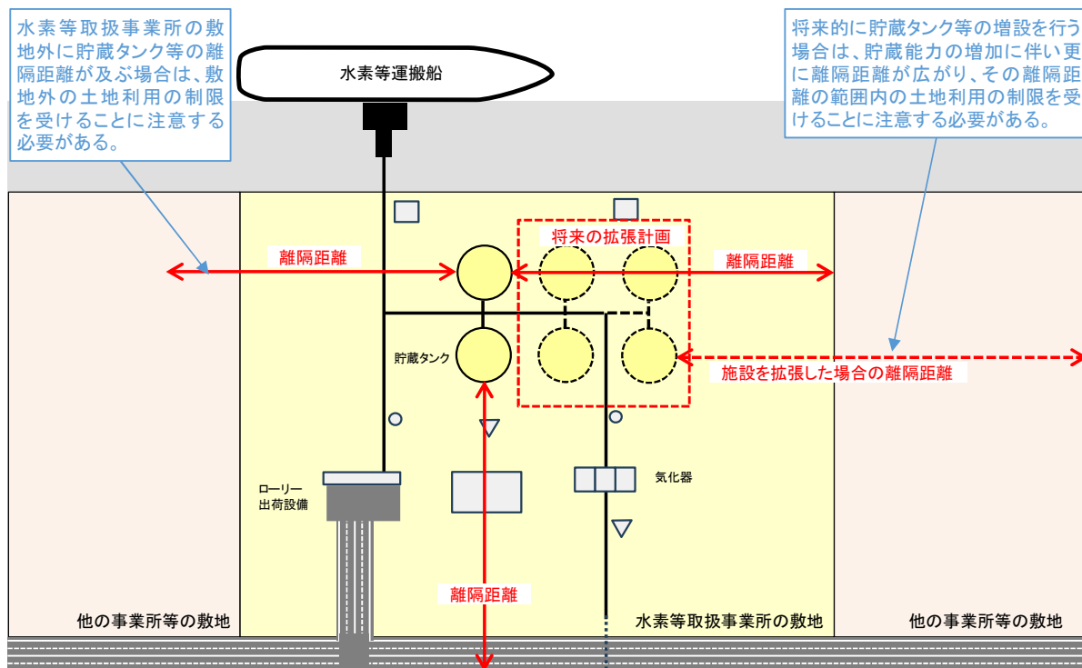
図-5.9 離隔距離の範囲内の土地利用が水素等の受入拠点に影響を及ぼす場合のイメージ
