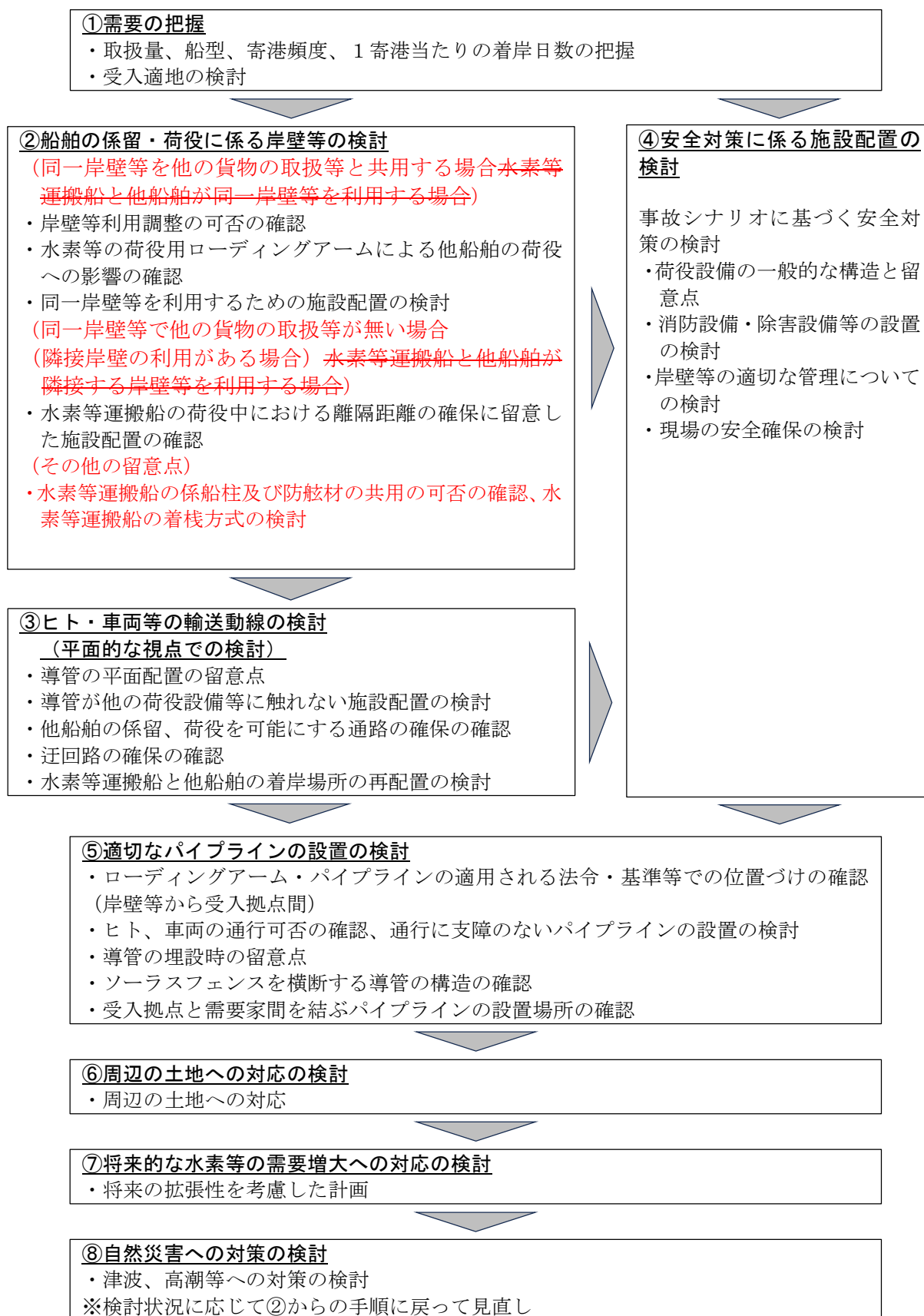
図-4.1 想定される水素等受入拠点の計画に係る手順
