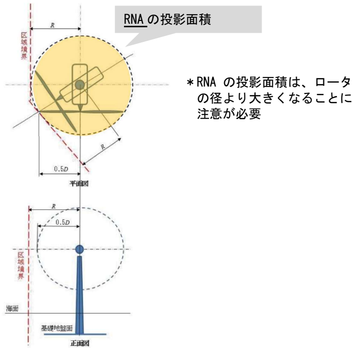
図－3 洋上風力発電設備における占用面積の考え方
