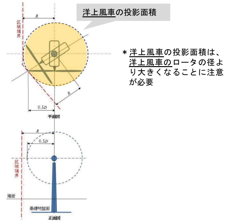
図－3 洋上風力発電施設における占用面積の考え方
