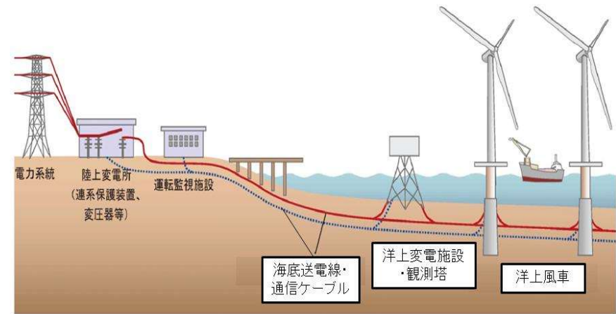
図-1 洋上風力発電施設等
