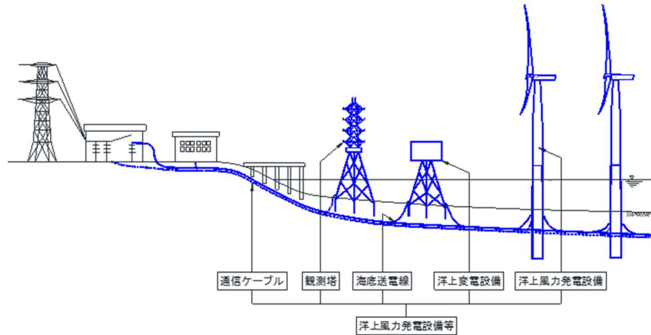
図-1 洋上風力発電設備等
