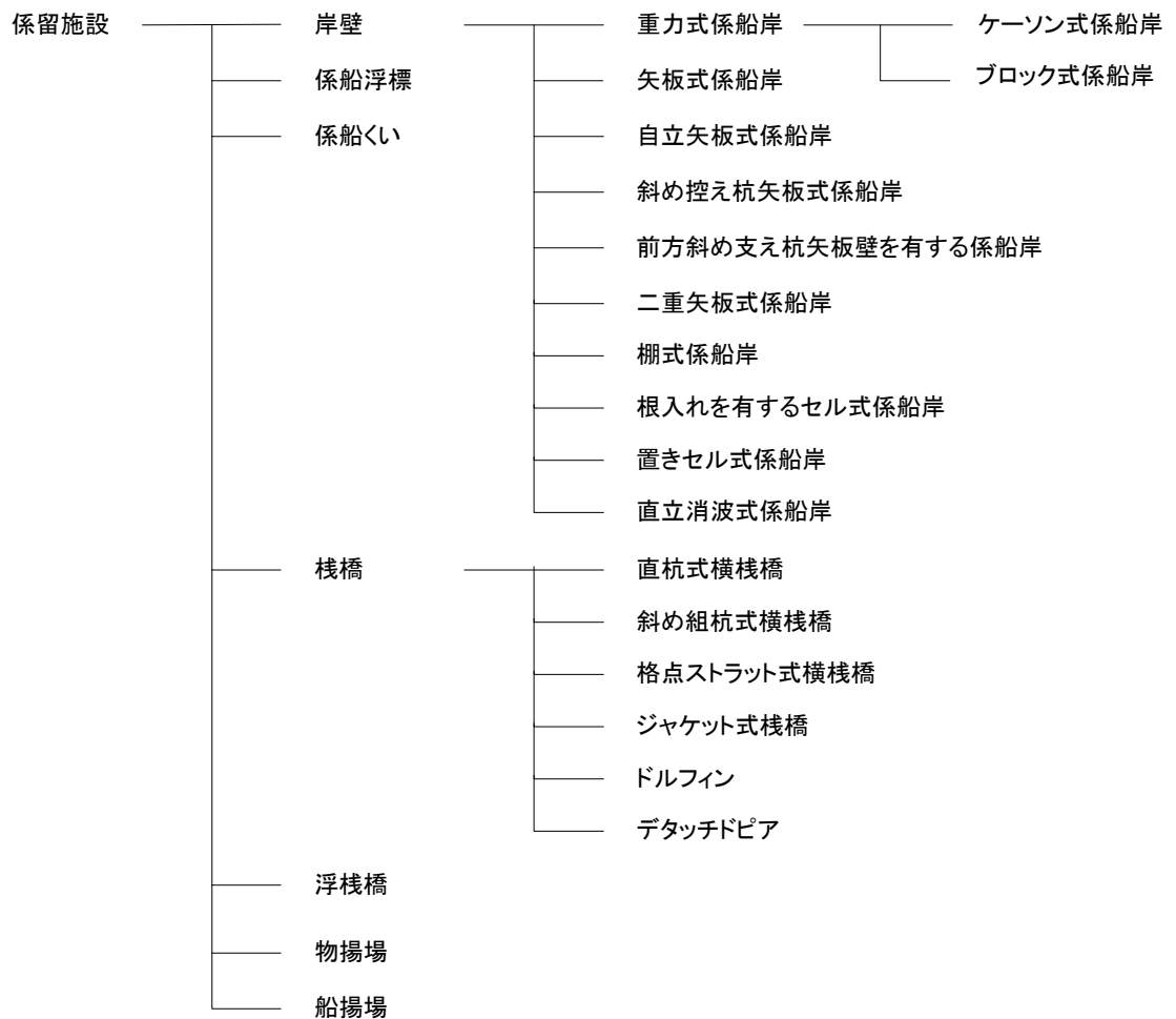
附図-3.1 係留施設の種類及び代表的な構造形式
