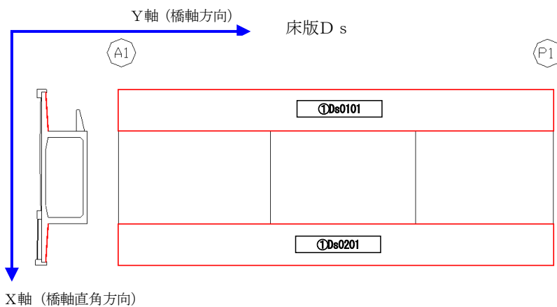
附図-4.5 床版に対する座標系
