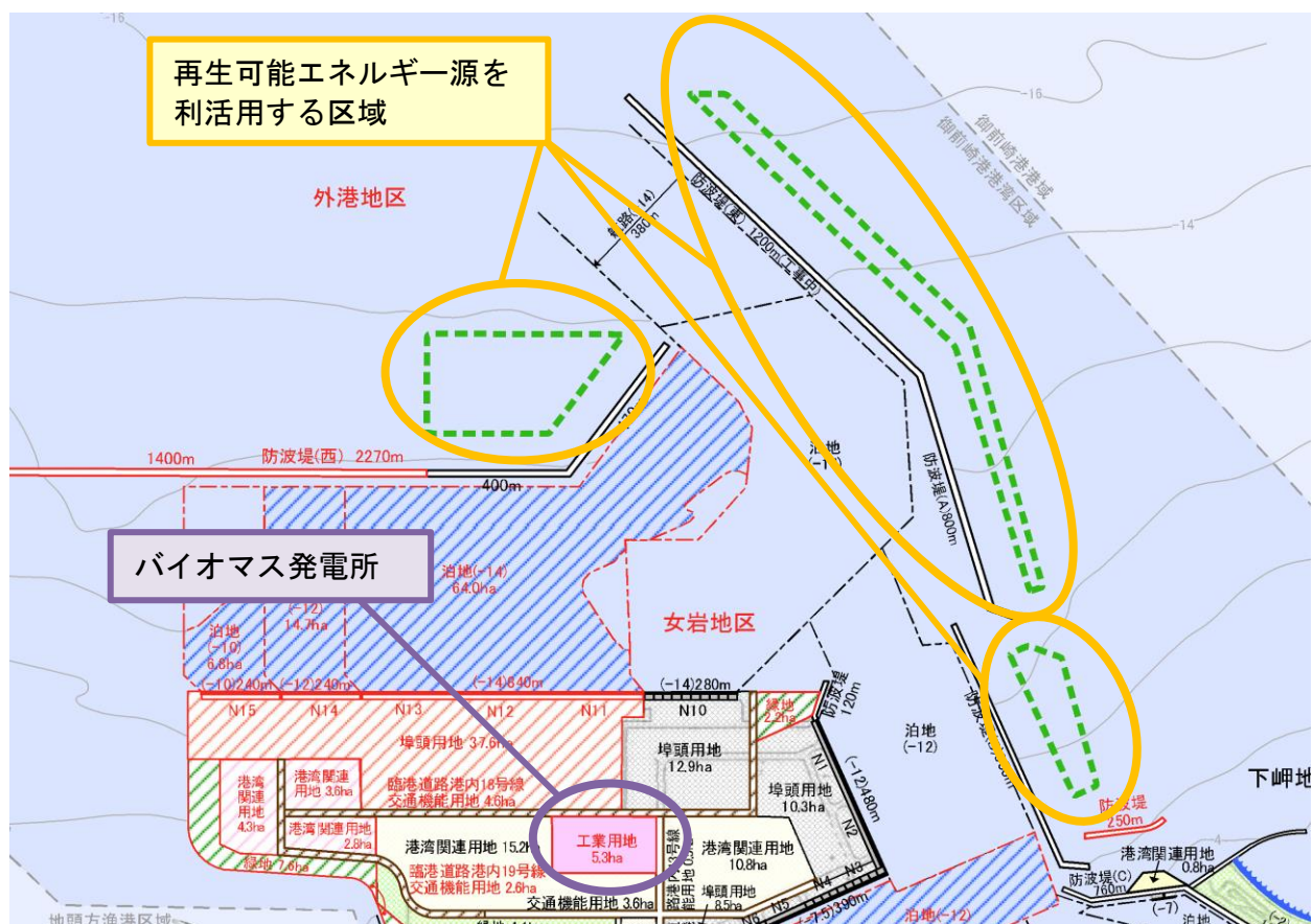
図４ 御前崎港港湾計画図（R3.2軽易な変更）
