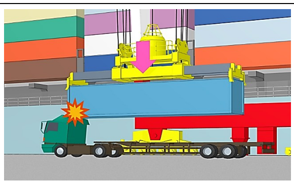
エプロン部でのシャーシとの接触
