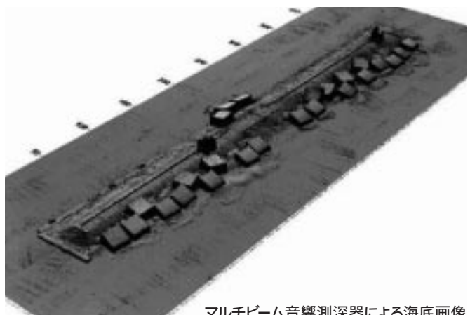
北海道函館港島防波堤の被災( 台風18号 )
