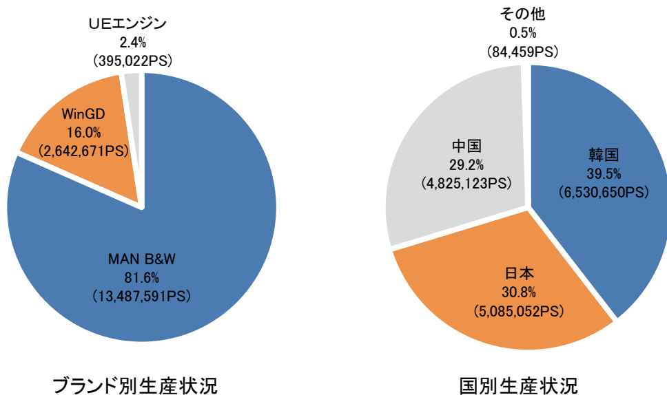
【図表 2-3】 2ストロークディーゼル機関のブランド・国別生産状況
