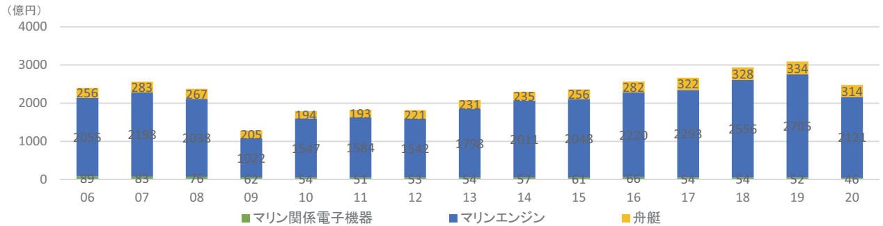
【図表2-5】 舟艇工業における総出荷額の推移
