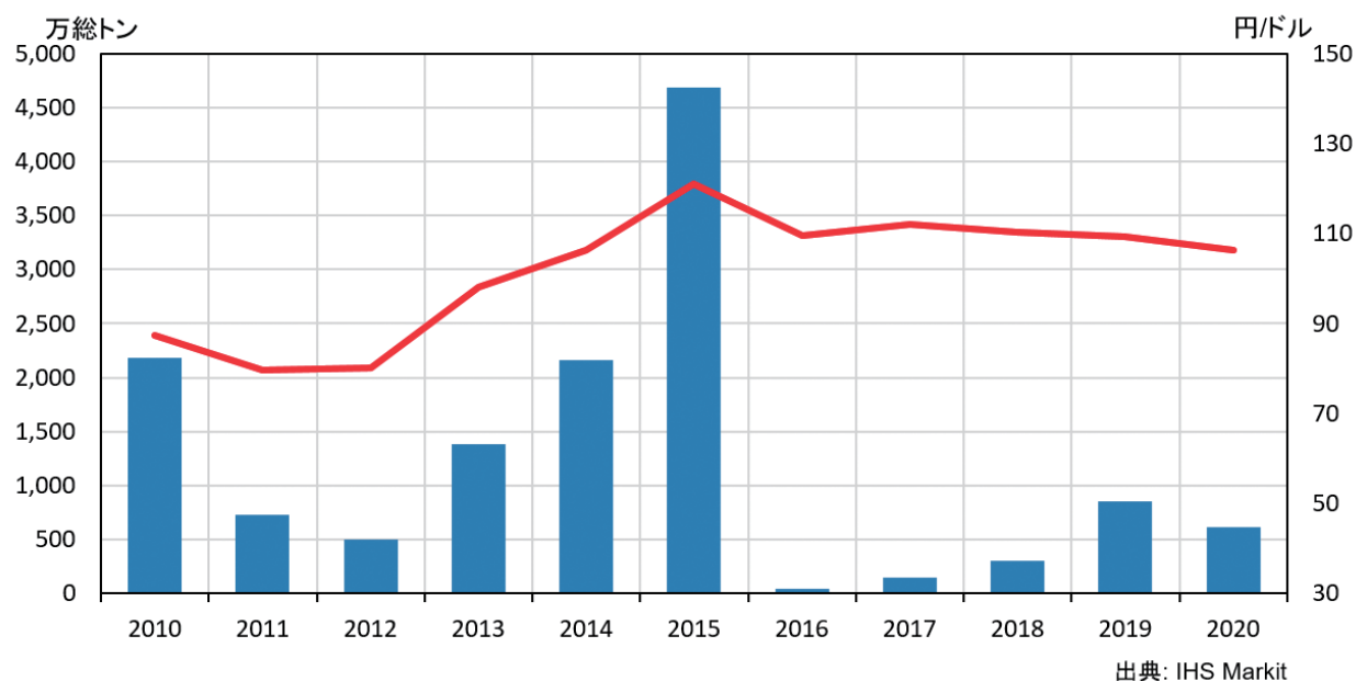
【図表2-2】我が国造船業の手持ち工事量の推移
