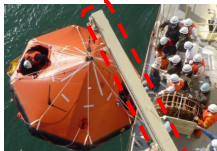
ダビット式進水装置
