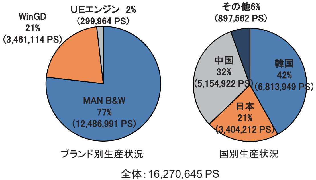
【図表 2-3】 2ストロークディーゼル機関のブランド・国別生産状況
