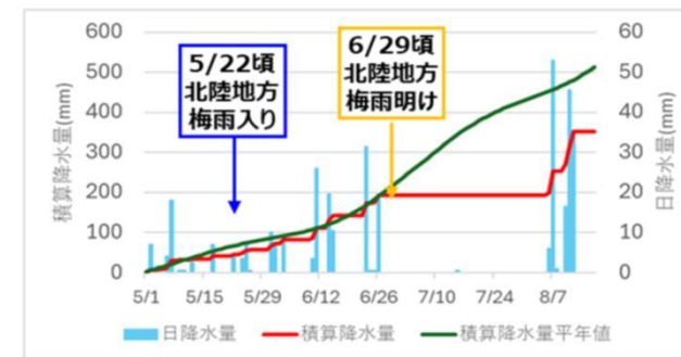
図-3 2025年5月から8月上旬にかけての新潟県高田の降水量の状況
