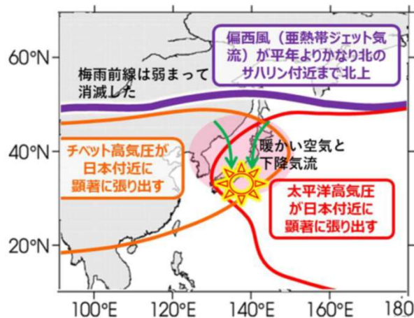
図-1 大規模な大気の流れの特徴とその天候への影響のイメージ(7月)
