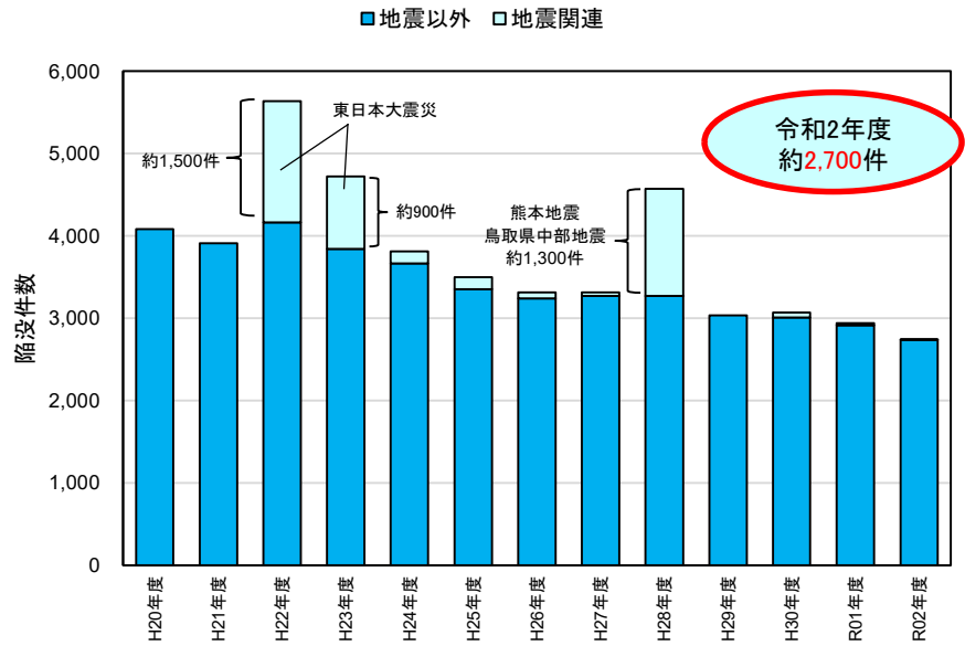
参考 3-8-4 下水道管路施設に起因した道路陥没件数の推移（令和2年度末）
