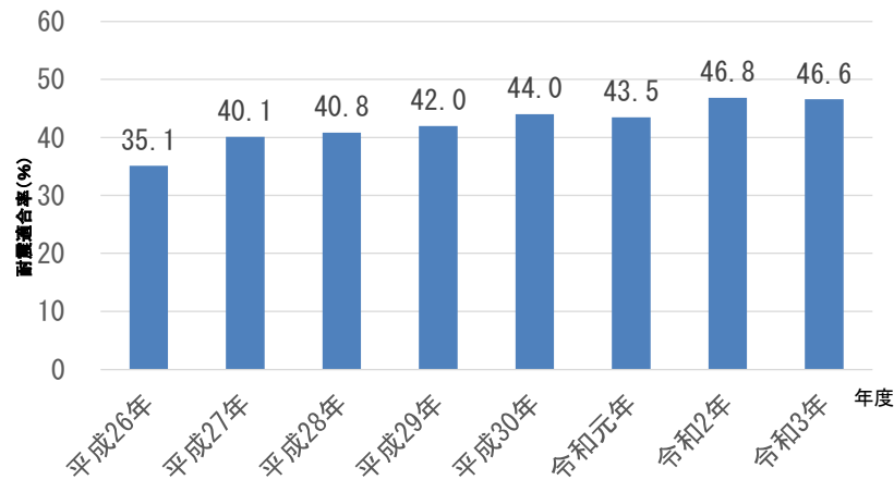
参考3-8-2 工業用水道施設の基幹管路の耐震化適合率
