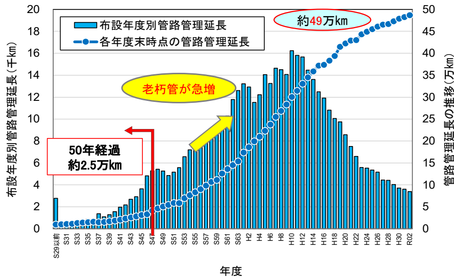
参考 3-8-3 下水道管路施設の年度別管理延長（令和2年度末）
