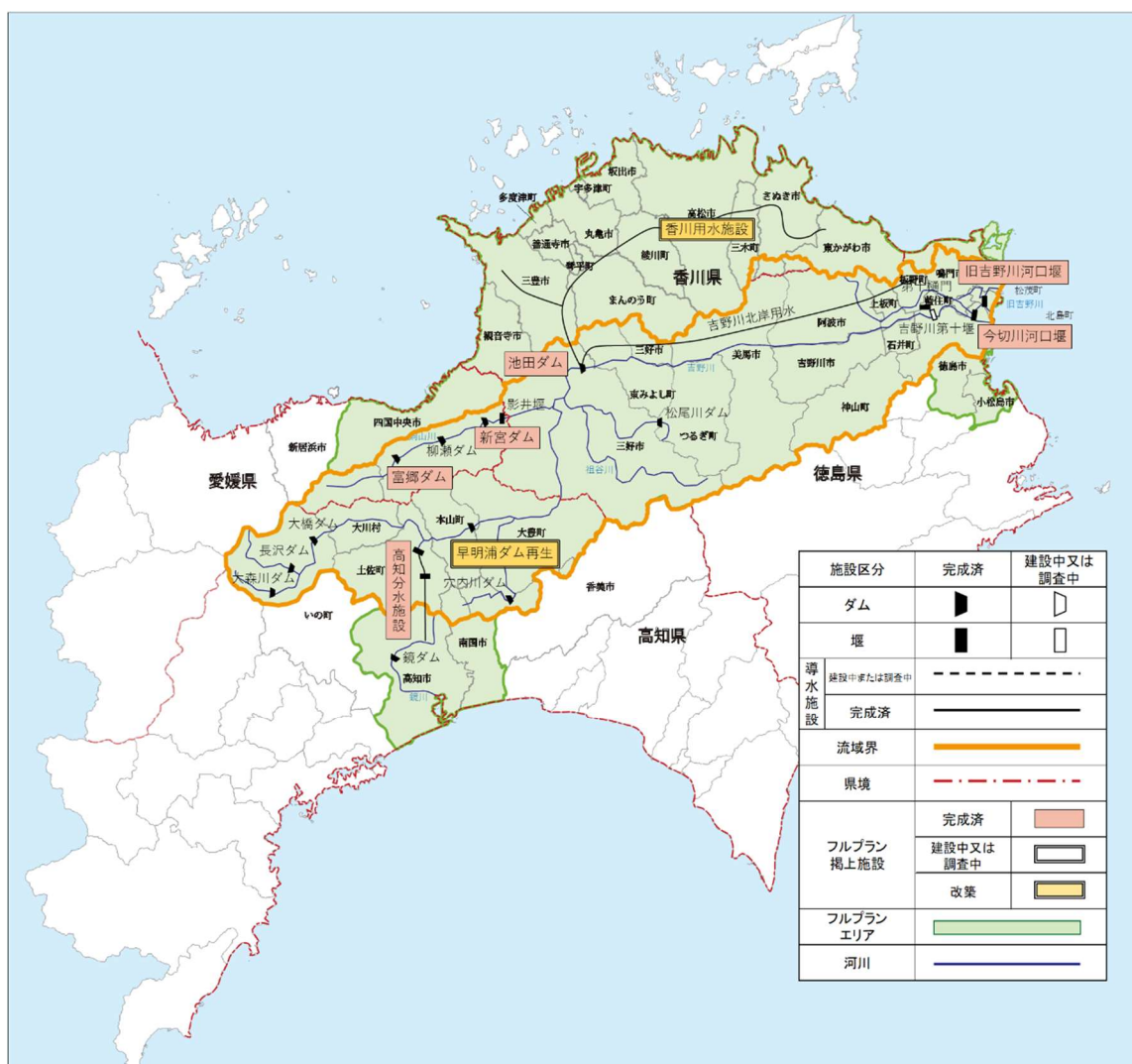
参考3-1-13 吉野川水系における水資源開発事業の位置図
