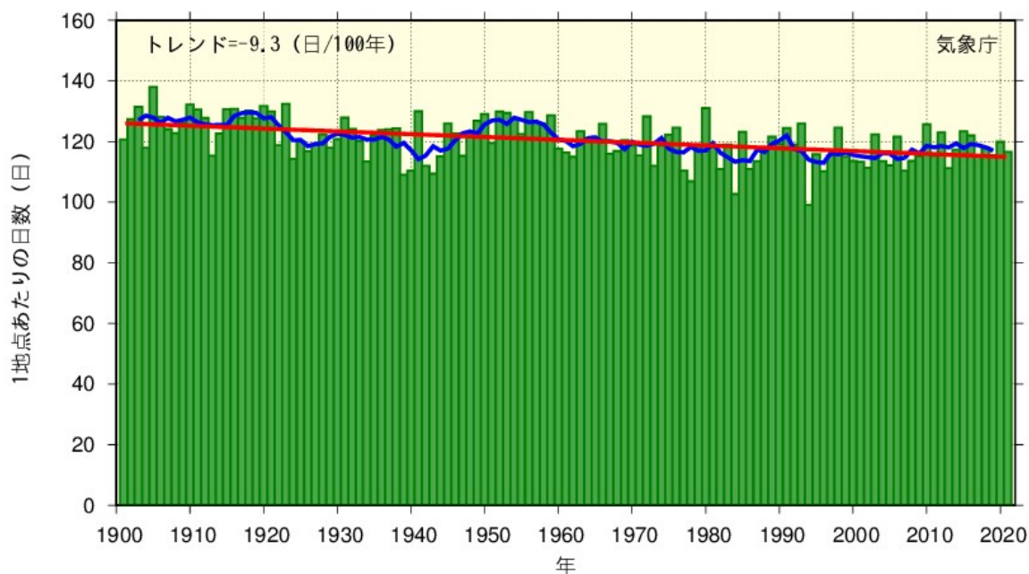
参考3-5-2 我が国の日降水量1.0mm以上の年間日数の経年変化
