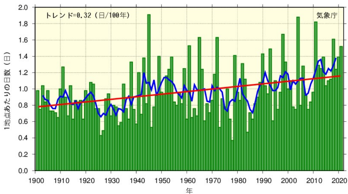
参考3-5-1 我が国の日降水量100mm以上の年間日数の経年変化
