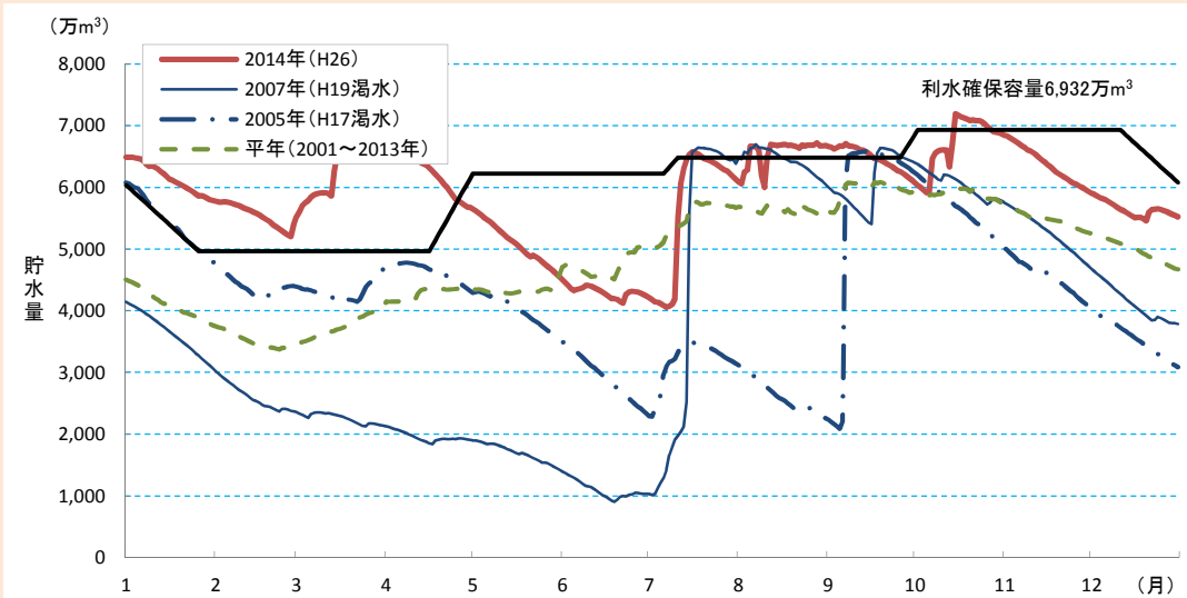
図4-8-15 銅山川3ダム（吉野川水系）貯水量図
