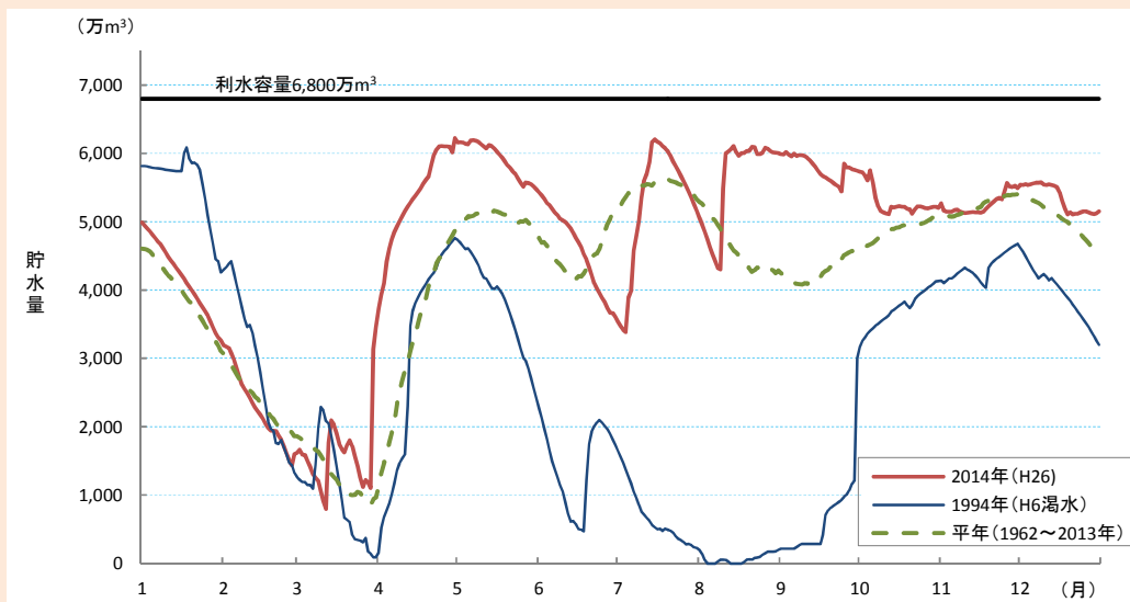
図4-8-9 牧尾ダム（木曽川水系）貯水量図
