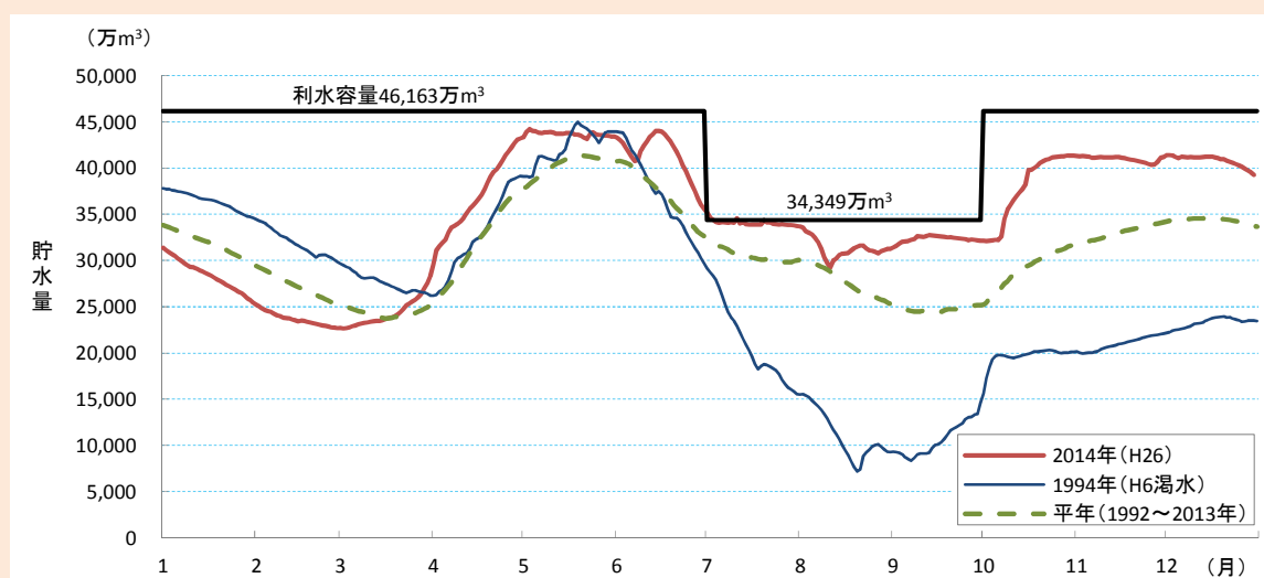
図 4-8-5 利根川上流 8 ダム貯水量図
