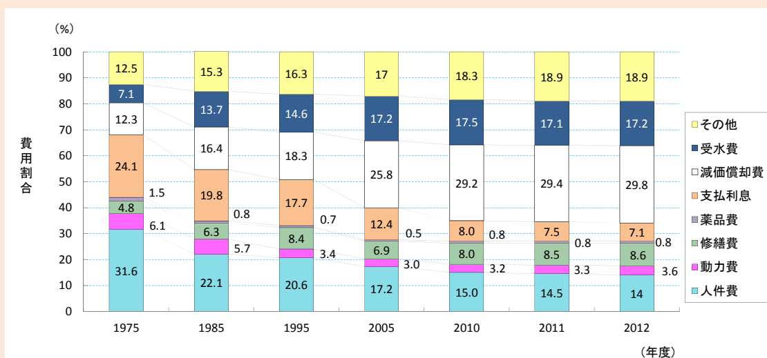
図4-1-20 上水道事業の費用内訳の推移
