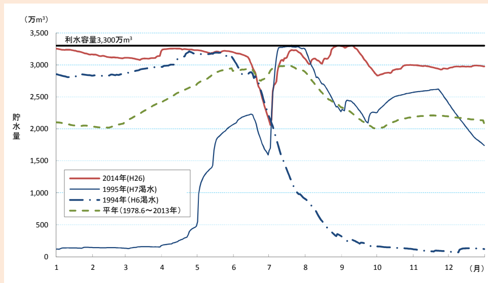
図4-8-17 江川ダム・寺内ダム（筑後川水系）2ダム貯水量図
