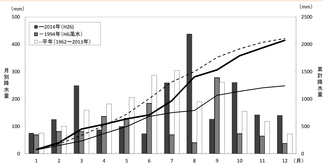
図4-8-8 降水の状況（牧尾ダム地点）
