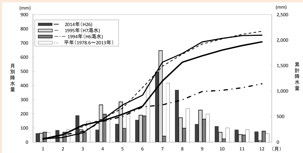
図4-8-16 降水の状況（江川ダム・寺内ダム上流域平均）
