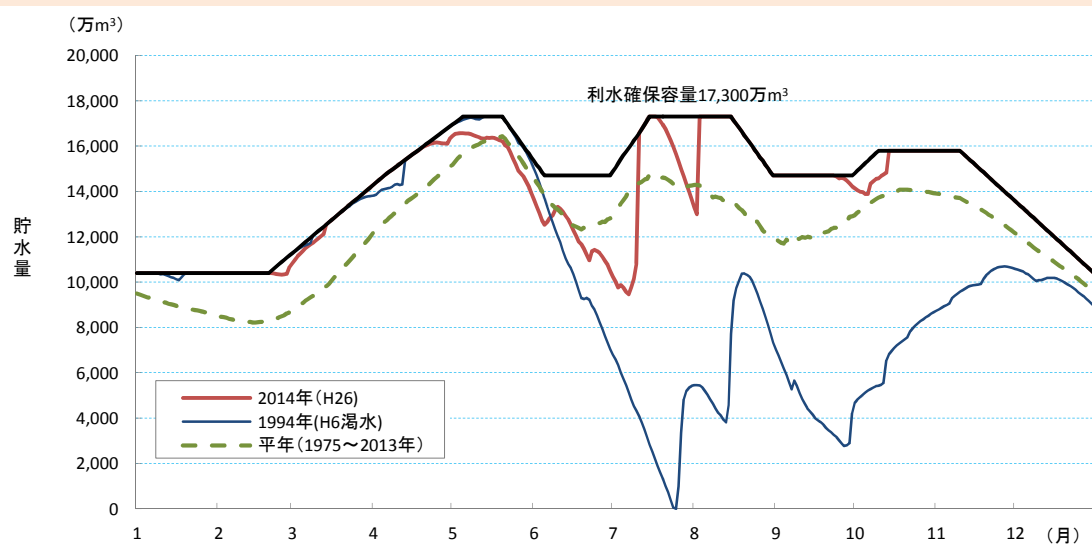
図4-8-13 早明浦ダム（吉野川水系）貯水量図
