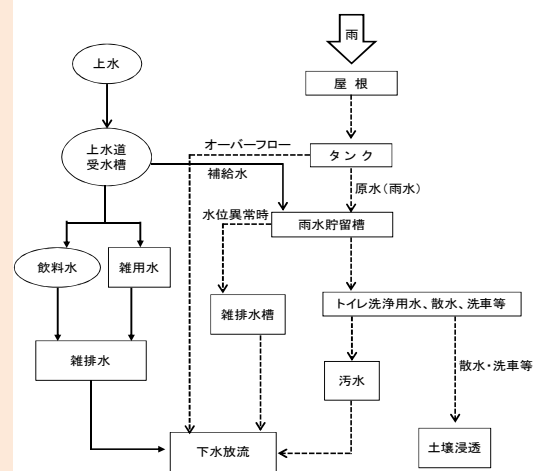
図4-2-2 雨水利用システム例
