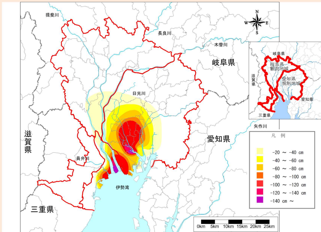
図 4 - 3 - 3 濃尾平野地盤沈下防止等対策要綱対象地域及び累積沈下量
