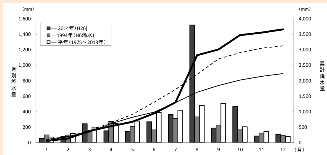
図4-8-12 降水の状況（早明浦ダム上流域）
