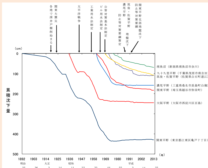
図4-3-1 代表的地域の地盤沈下の経年変化
