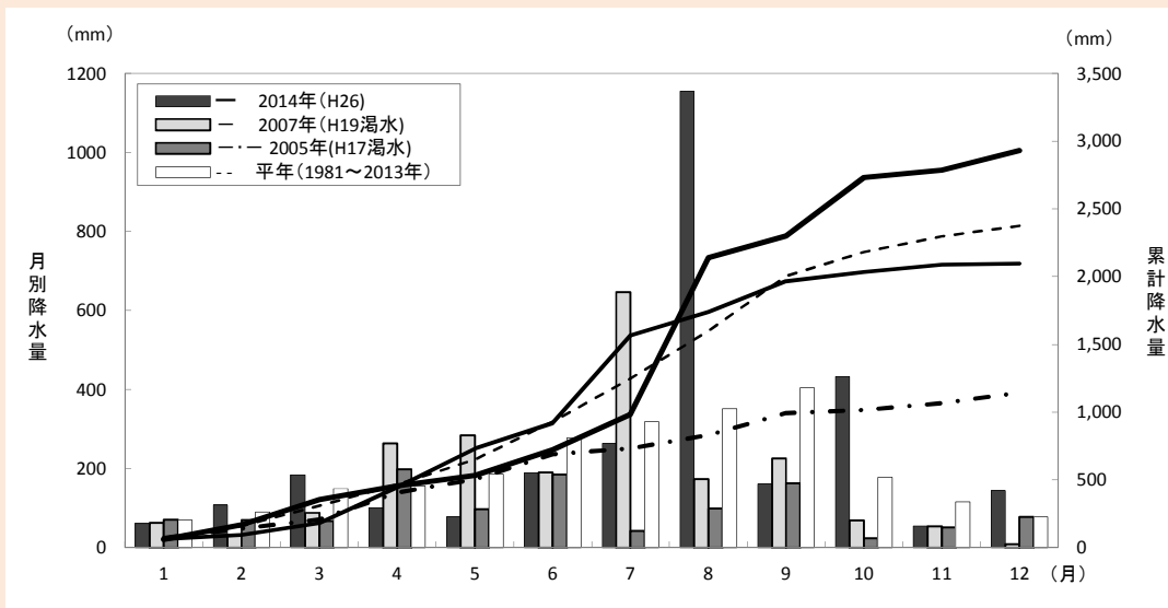
図4-8-14 降水の状況（新宮ダム上流域）
