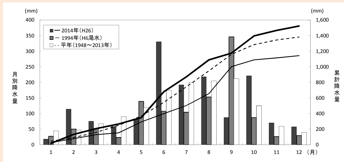
図 4-8-4 降水の状況（利根川上流域）
