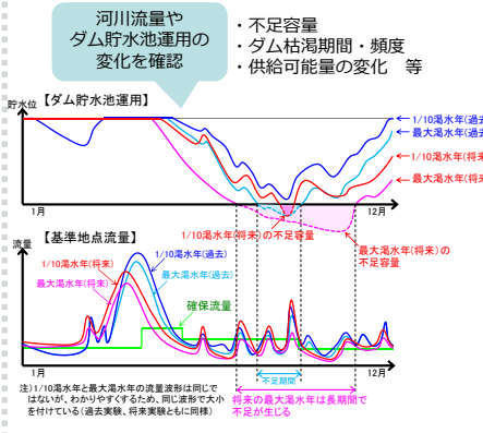
図 4.12 貯水池運用及び基準地点流量の評価結果のイメージ
