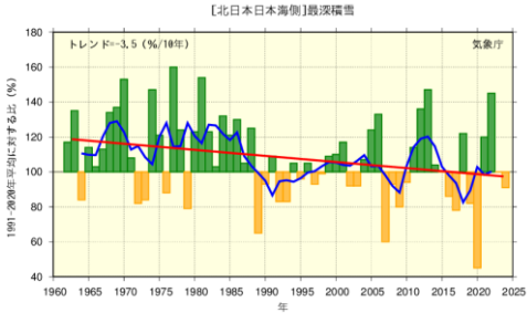
図 3.3 日本の年最深積雪の基準値に対する比率の経年変化（1962～2024年）及び全国及び地域別の年最深積雪の将来変化[1]
