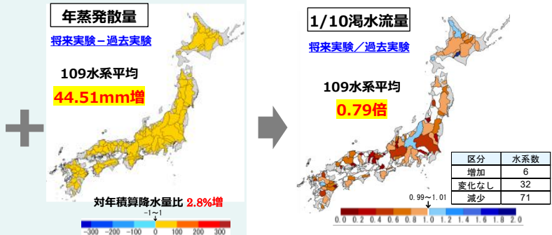
図 3.4 年蒸発散量の変化（将来実験－過去実験）[2]
