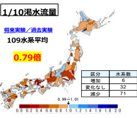
図 3.5 河川流量の変化（将来実験／過去実験）[2]
