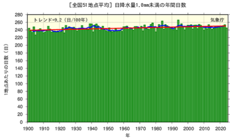
図 3.1 無降水日（日降水量1.0mm未満）の年間日数の経年変化（1901～2024）[1]
