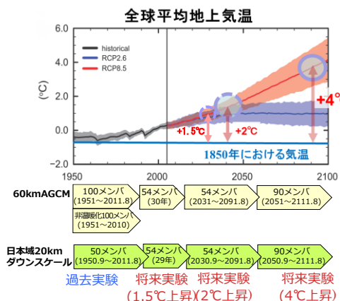
図 4.6 d4PDFの実験デザイン
