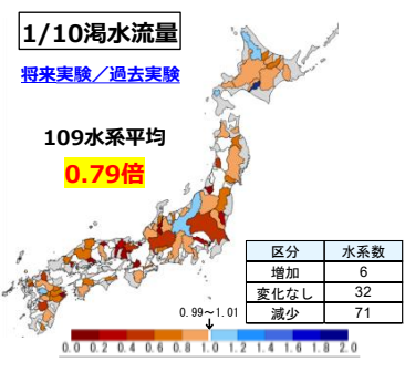
図 3.5 河川流量の変化（将来実験／過去実験）[2]
