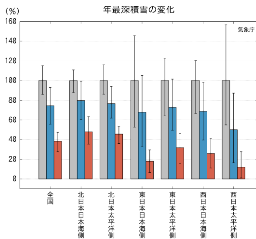
図 3.6 日本の年最深積雪の基準値に対する比率の経年変化（1962～2024 年）及び全国及び地域別の年最深積雪の将来変化 [1]
