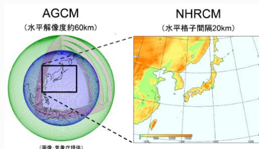
図 2.2 MRI-AGCM3.2 と NHRCM
