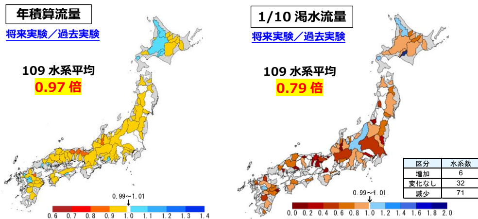
図 3.8 河川流量の変化（将来実験／過去実験） [2]
