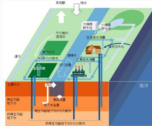
図 4.15 全球水資源モデル H08 における水循環・水利用・水管理の模式図
