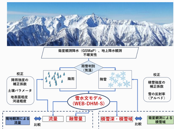
図 4.16 WEB-DHM-S の構築フロー
