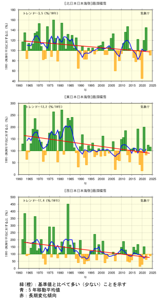
図 3.6 日本の年最深積雪の基準値に対する比率の経年変化（1962～2024 年）及び全国及び地域別の年最深積雪の将来変化 [1]
