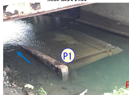
橋脚被災状況
