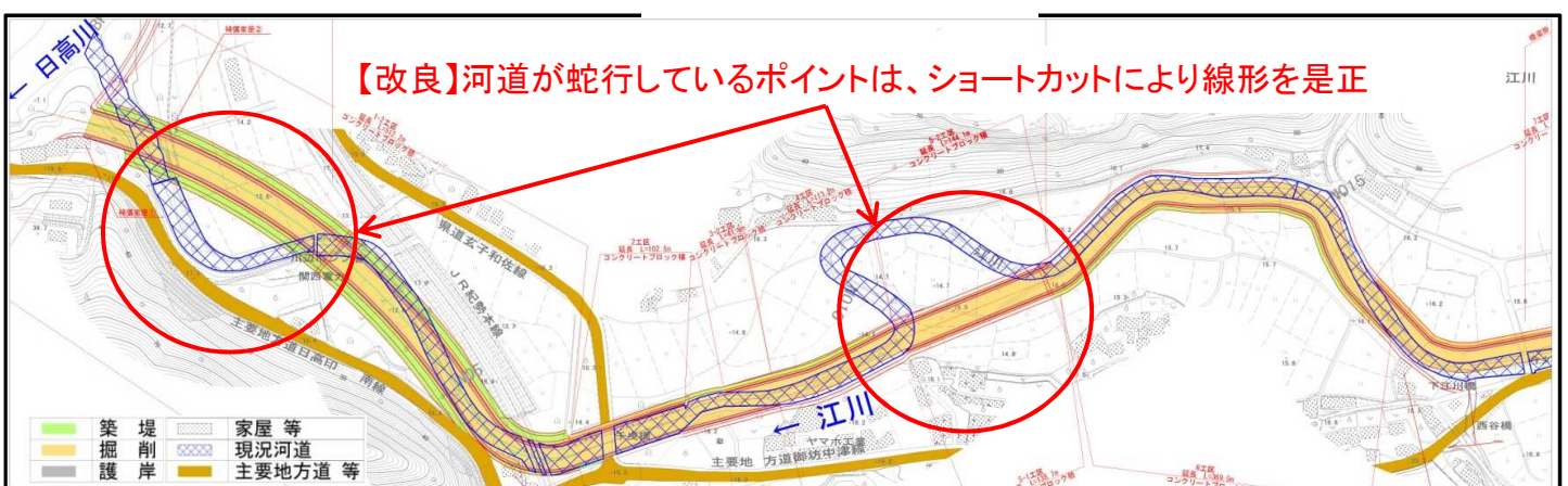
平面図 (下流区間)
