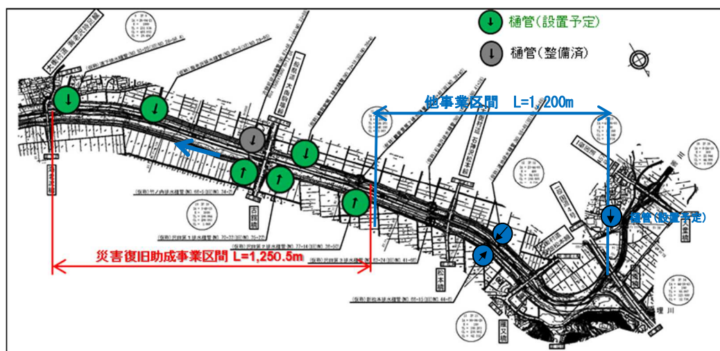
平面図
