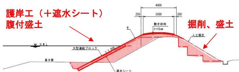
横断図（右岸）
