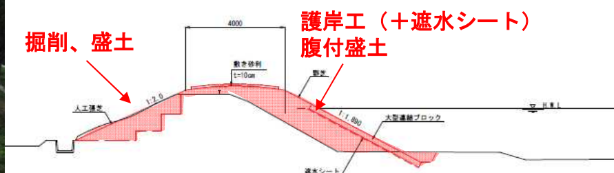
横断図（左岸）
